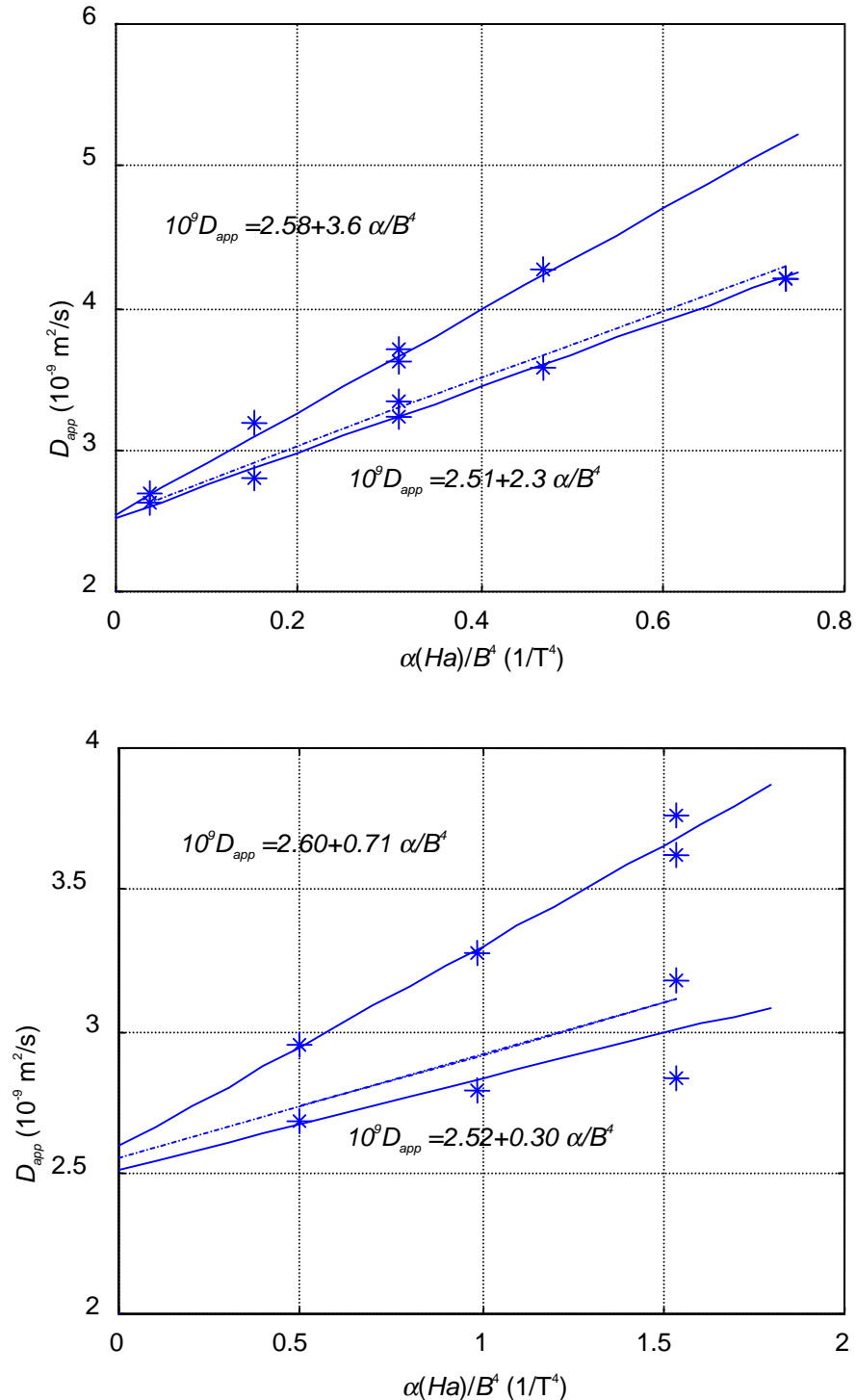
Figure 5.2 : Résultats expérimentaux sur SnIn (1%), la température moyenne est de 275^\circ\text{C} .
