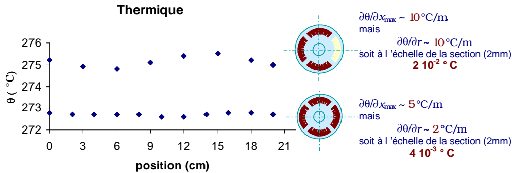
Figure 5.4 : Profils de température pour les deux expériences sur l'influence des gradients radiaux de températures.
