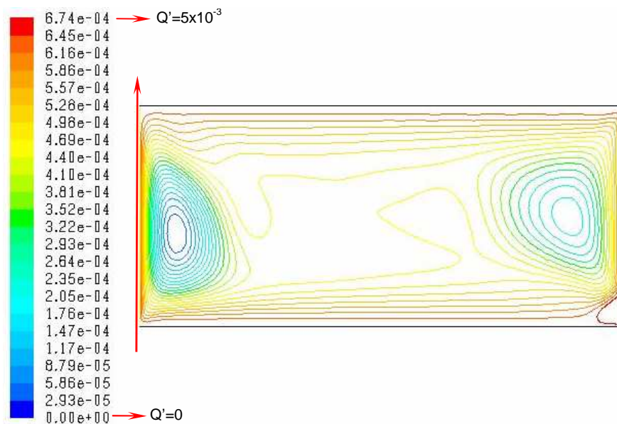
Figure 6.5. Présentation des lignes de courant de l'écoulement en présence de champ magnétique B=0,3T ( Nc = 3 \times 10^7 ). Ra \approx 10^{10}
