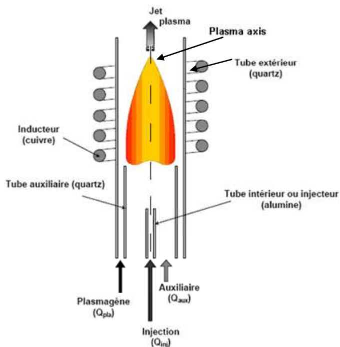
Figure VI-6: principe de fonctionnement d'une torche ICP.
