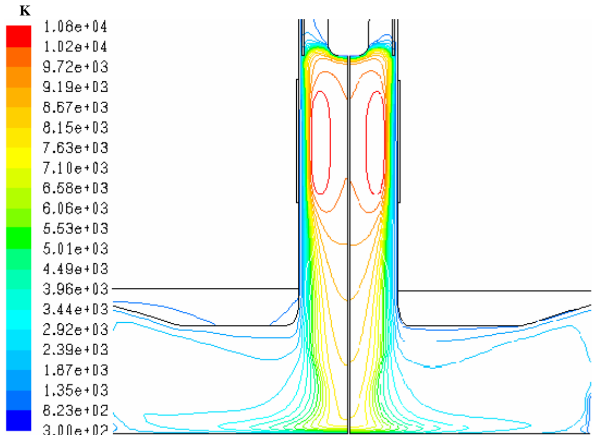
Figure III-10 : champ de température en fonction de l'émissivité des parois : (a, gauche) : \varepsilon = 1 partout. (b, droite) : \varepsilon adapté au matériau (Tableau III-2).
