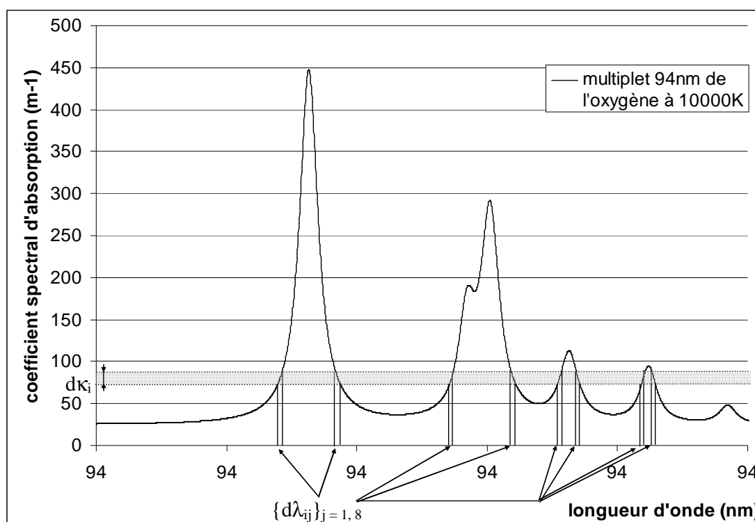
Figure IV-15 : illustration de la méthode de regroupement des intervalles spectraux proposée par Modest pour le multiplet O 94nm dans un milieu isotherme.
