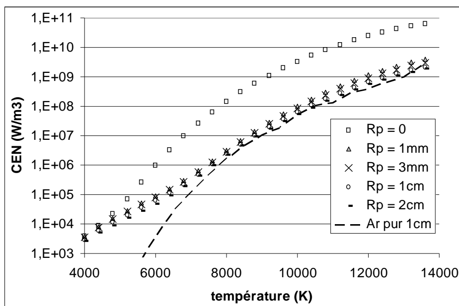
Figure IV-9 : coefficient d'émission nette d'un mélange 95%Ar, 5% O_2 en volume en fonction de T et pour différents rayons plasma. Les valeurs obtenues en argon pur sont rappelées pour faciliter la comparaison.
