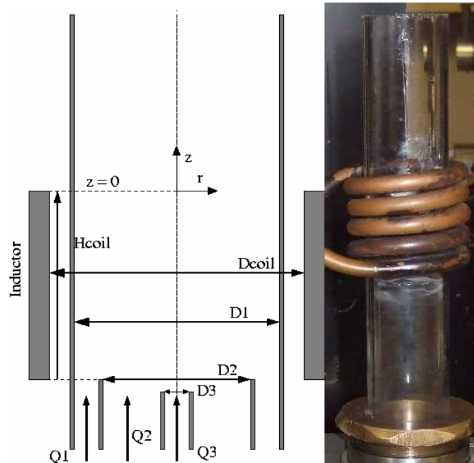
Figure III-1 : schéma de principe des torches plasma (gauche). Photo d'une torche d'analyse (droite).
