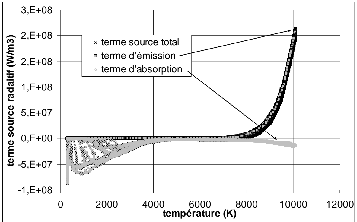
Figure V-16 : composantes du terme source radiatif calculé avec le modèle P1 : perte de chaleur en positif (afin de respecter le format des courbes CEN), chauffage radiatif en négatif.
