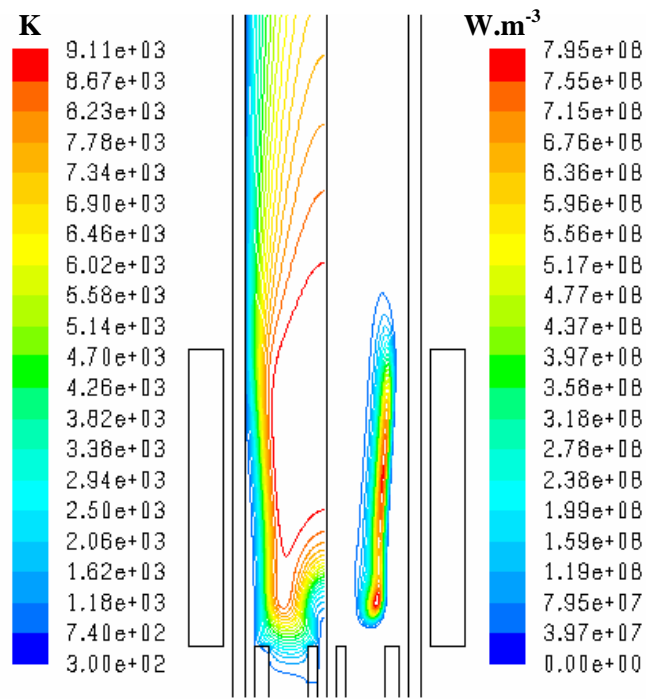
Figure VII-3 : résultats de la simulation de l'expérience de [Regt, 1995] : température (gauche) et puissance Joule (droite)
