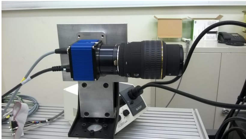
FIGURE 3.2 - Caméra Haute Résolution 16 mégapixels.
