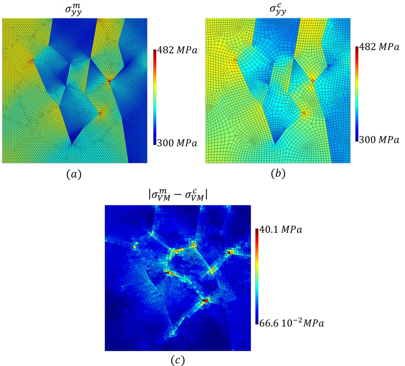
FIGURE 4.21 - Contrainte transversale au dernier pas de chargement obtenue par : le calcul par EF \underline{\sigma}_{yy}^m (a) et par l'identification \underline{\sigma}_{yy}^c (b) et la contrainte de Von Mises de l'erreur absolue (c).
