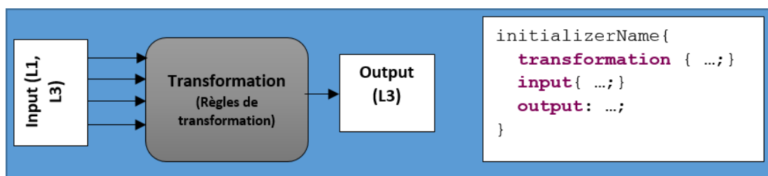
Figure 68. Les trois parties de la syntaxe concrète de L2
