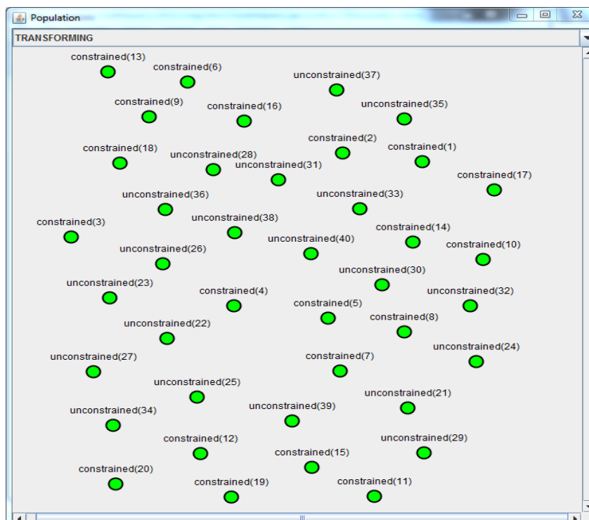
Figure 69. Génération graphique de l'état initial des prédateurs dans l'environnement
