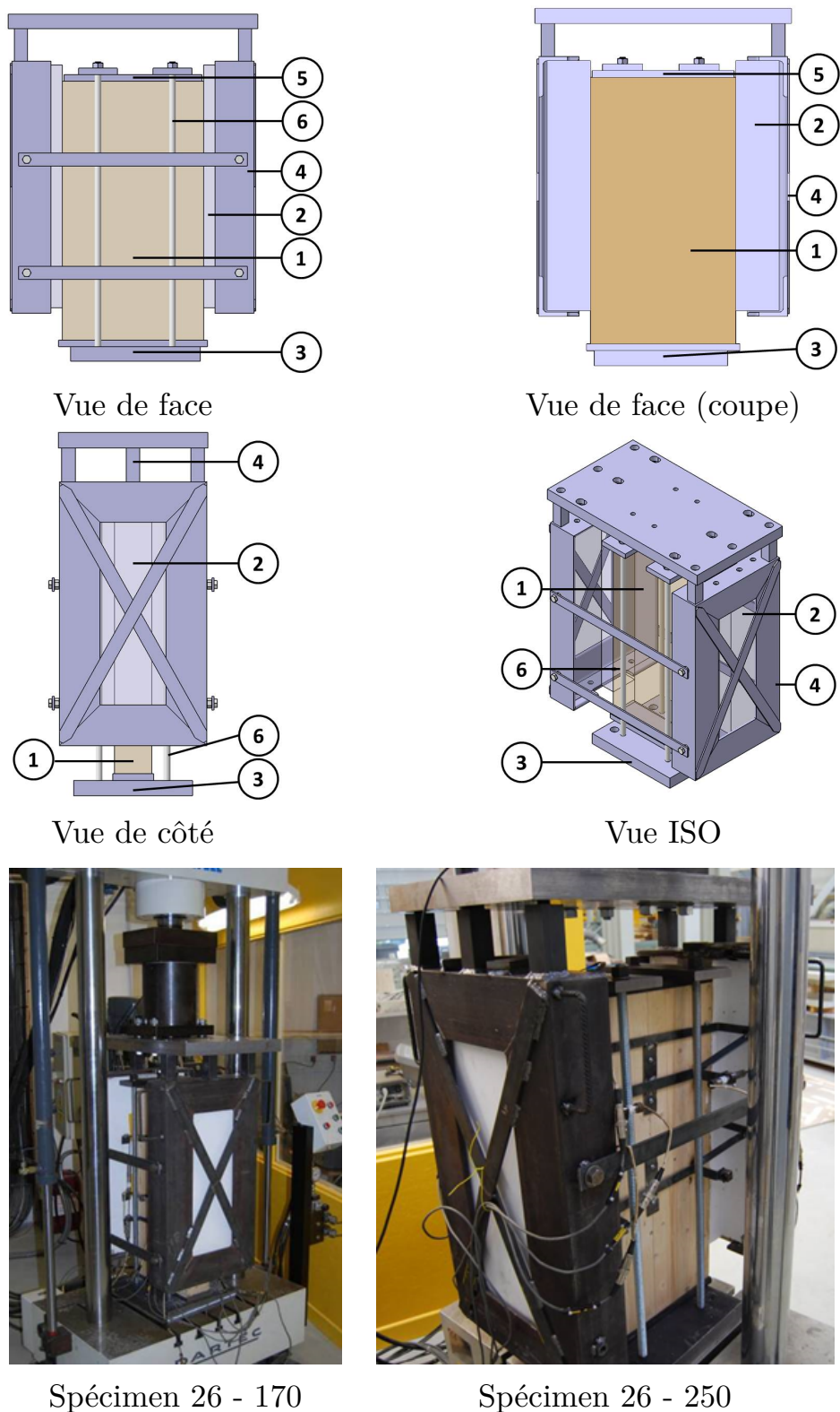
Figure 2.2 – Montage expérimental des essais Push-Out
