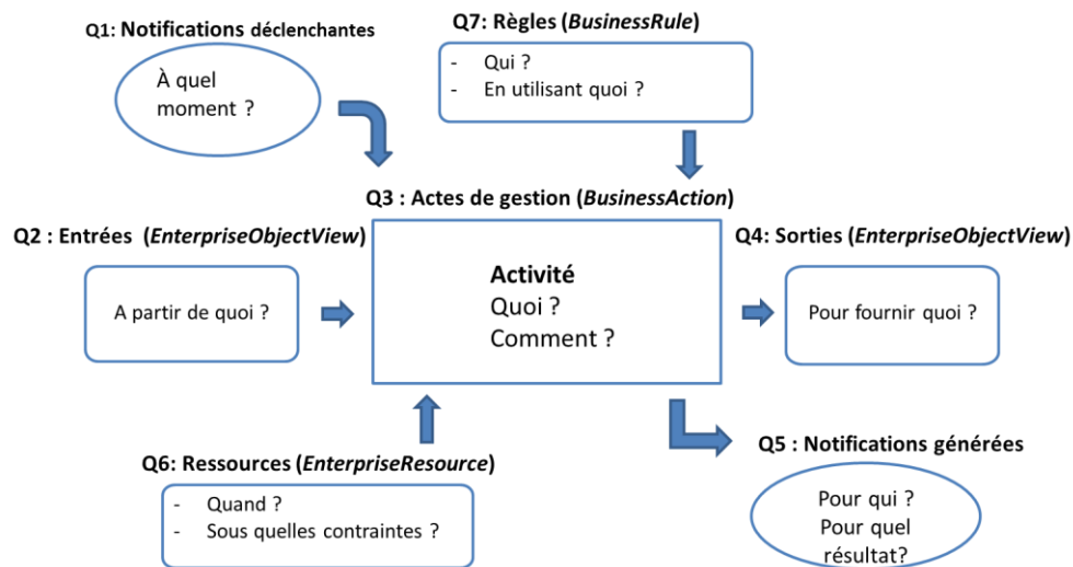
Figure 19. Questions intervenant dans la définition d'une activité.
