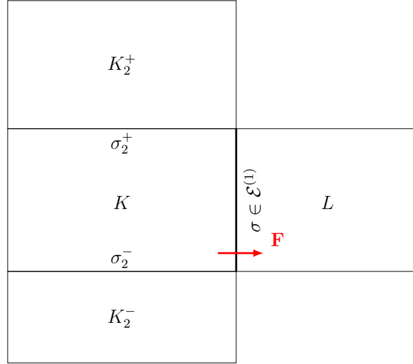
FIGURE 1.3 – Notations pour la construction du gradient sur maillage cartésien avec \mathbf{F} = (G_L - G_K)\mathbf{n}_{K,\sigma} .
