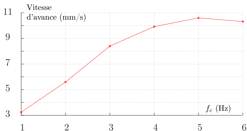
FIGURE 3.38 – Evolution de la vitesse d'avance en fonction de f_c .
