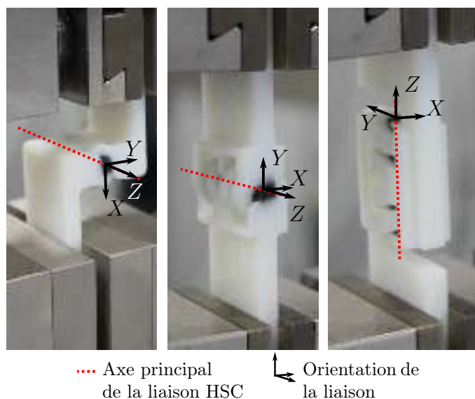
FIGURE 2.25 – Expérimentation pour la mesure des compliances secondaires.
