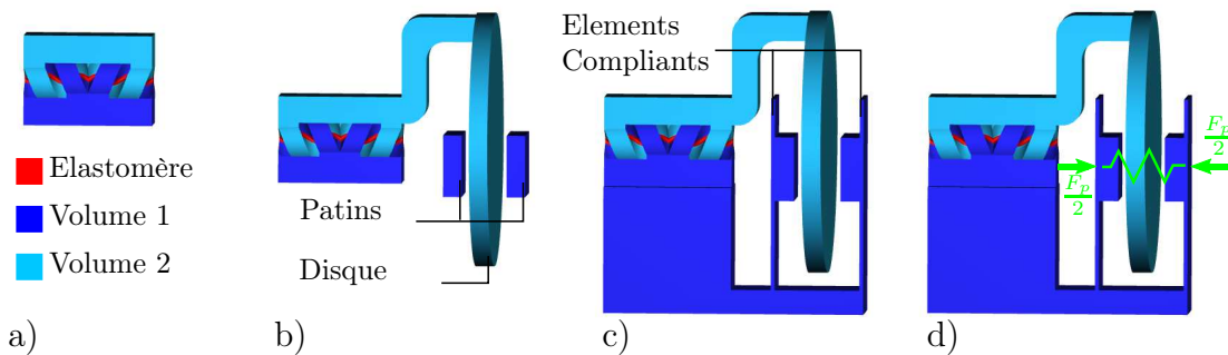
FIGURE 3.12 – Schéma de construction du système de freinage. a) Liaison compliant seule, b) Positionnement du disque et des patins, c) Ajout des deux éléments compliants, d) Ajout de la précontrainte.
