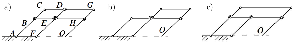
FIGURE 4.5 – a) Configuration de base d'un mécanisme parallélogramme. b) et c) Configurations dérivées.
