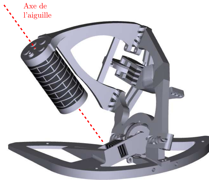
FIGURE 4.32 – Modèle CAO du troisième dispositif.
