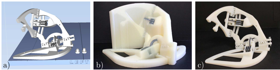
FIGURE 4.20 – Vues du deuxième dispositif : a) durant le pré-traitement, b) après fabrication, c) après post-traitement.
