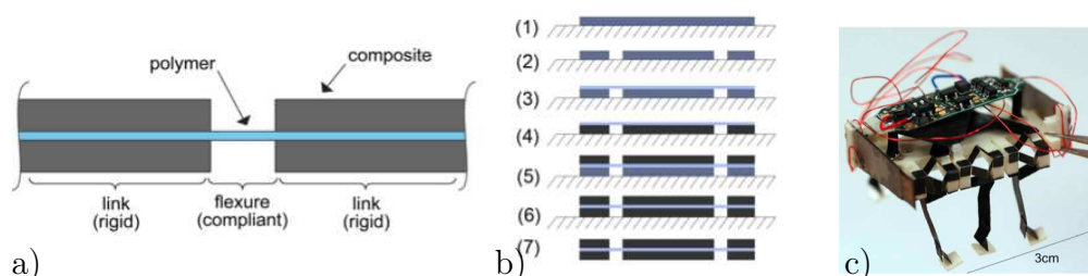
FIGURE 1.13 – a) Réalisation d'une liaison compliant. b) Principe du procédé SCM. c) Exemple de mécanisme spatial produit avec le procédé SCM.
