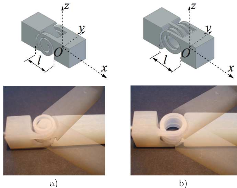
FIGURE 2.19 – Liaisons développées par Berselli et al. [Berselli 2011]. a) Liaison SPIR. b) Liaison HEL.
