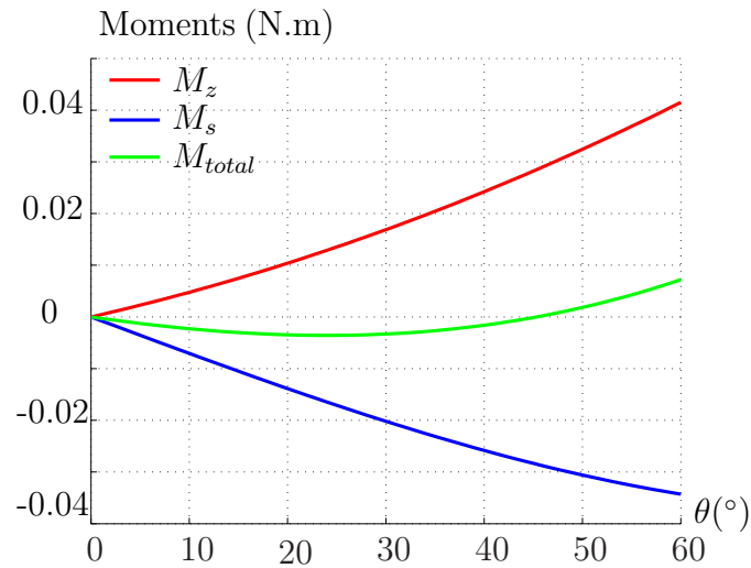
FIGURE 3.7 – Evolution par simulation des moments M_z , M_s et M_{total} en fonction de l'angle \theta .
