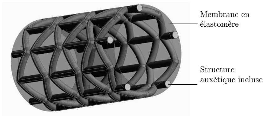
FIGURE 3.21 – Vue CAO de la membrane auxétique.
