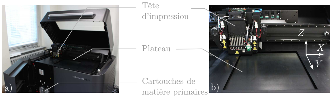
FIGURE 2.2 – a) Imprimante 3D Connex 350. b) La tête d'impression.
