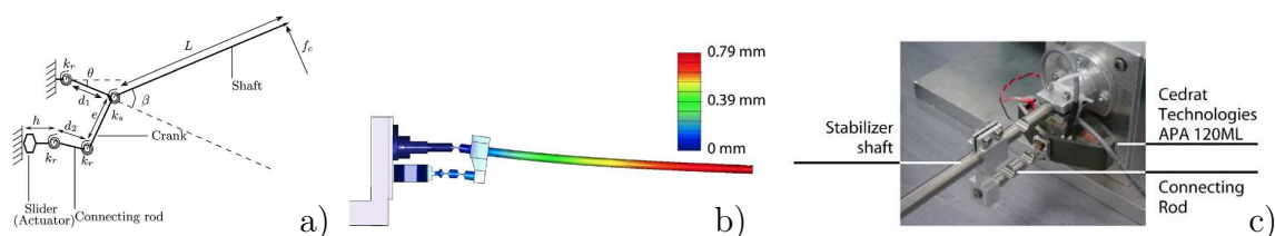
FIGURE 1.18 – Approche cinématique ([Bachta 2011]) : a) Modèle PRBM du mécanisme. b) Modèle CAO. c) Système réel.
