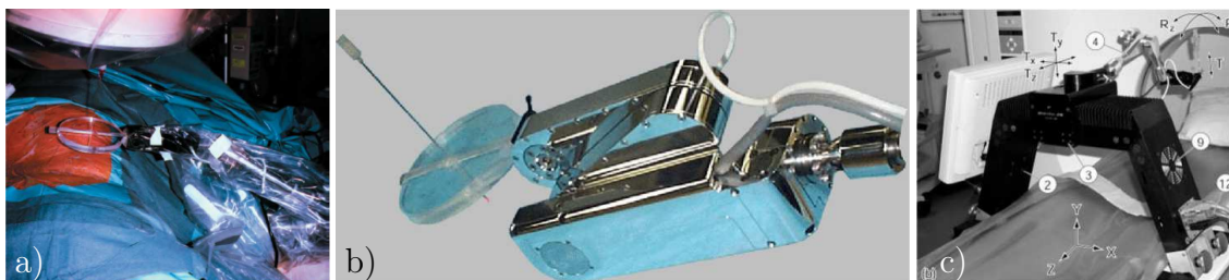
FIGURE 1.5 – a) Système d'insertion d'aiguille PAKY monté sur un bras passif. b) Système d'insertion d'aiguille PAKY monté sur un mécanisme RCM motorisé. c) Système AcuBot.
