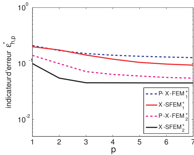
FIG. 3.28 – Exemple 1 : convergence de l'erreur \varepsilon_{h,p}^* , basée sur norme énergétique, en fonction de p pour h = 0.09 .
