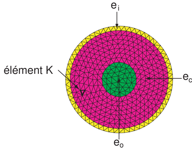
FIG. 2.30 – Exemple 3 : maillage X-SFEM avec états des éléments.
