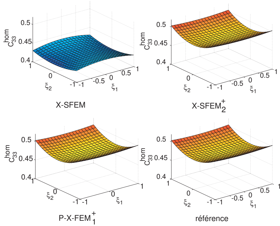
FIG. 3.34 – Exemple 2 : surfaces de réponse de la composante C_{33}^{\text{hom}} obtenue avec X-SFEM, X-SFEM _2^+ , P-X-FEM _1^+ et la solution de référence X-FEM ^+ .
