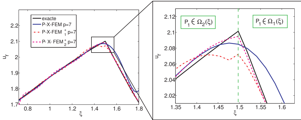
FIG. 3.27 – Exemple 1 : surfaces de réponse du déplacement radial en P_1 obtenues avec les solutions P-X-FEM, P-X-FEM _1^+ et P-X-FEM _2^+ .
