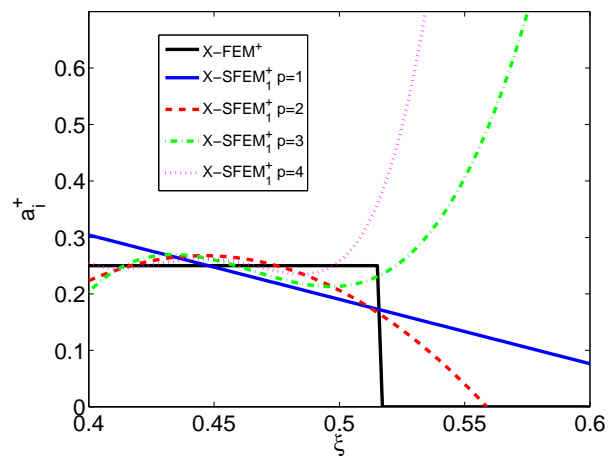
FIG. 3.9 – Exemple de référence : surfaces de réponse d'un degré de liberté enrichi obtenus avec X-SFEM 1 + pour différents ordres de chaos polynomial p ; maillage 2 .
