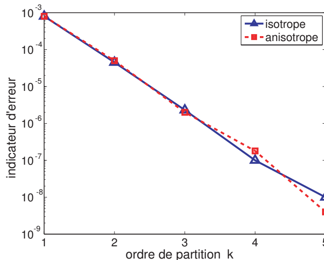
FIG. 2.15 – Exemple 1 : convergence de l'indicateur d'erreur global \varepsilon^k en fonction de k pour les procédures isotrope et anisotrope.
