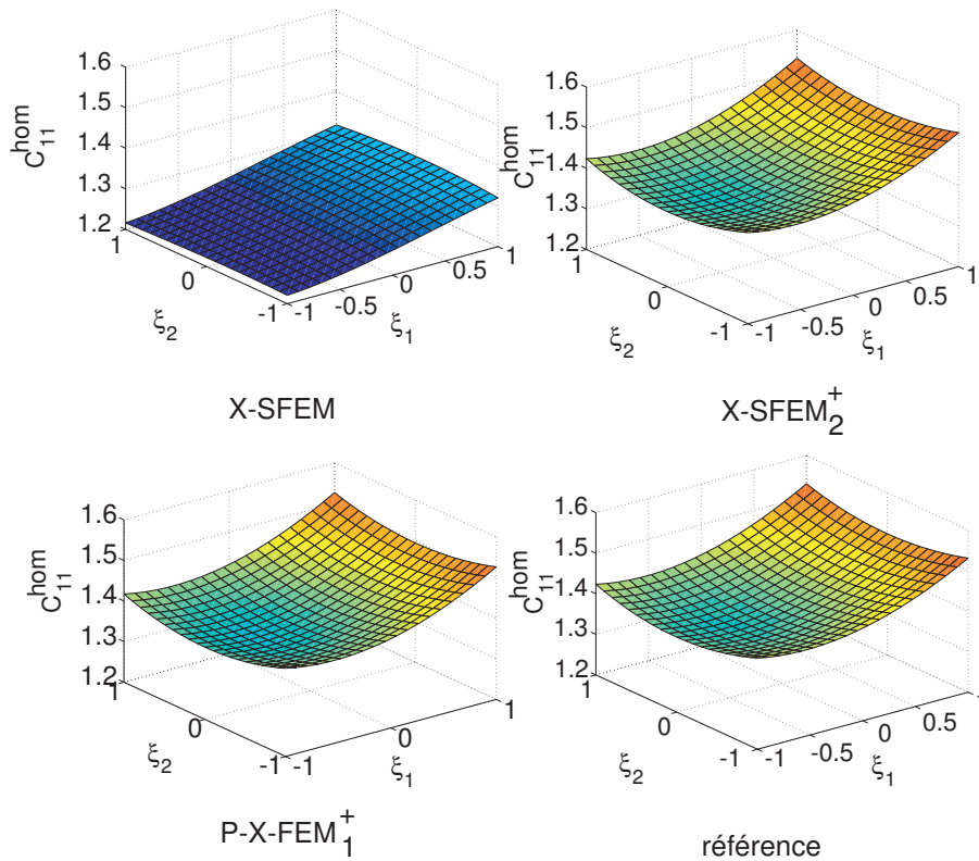
FIG. 3.33 – Exemple 2 : surfaces de réponse de la composante C_{11}^{hom} obtenue avec X-SFEM, X-SFEM _2^+ , P-X-FEM _1^+ et la solution de référence X-FEM ^+ .
