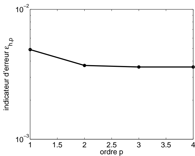
FIG. 2.34 – Exemple 3 : convergence de \varepsilon_{h,p} en fonction de p pour h = 0.18 .
