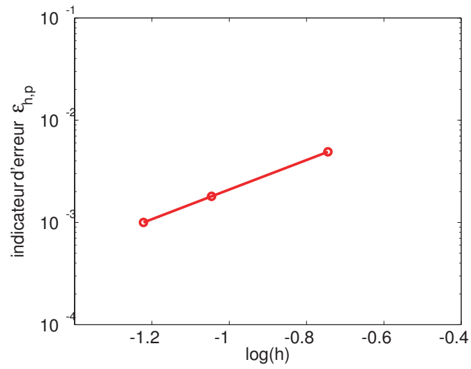
FIG. 3.24 – Exemple 1 : convergence en fonction de h de l'erreur \varepsilon_{h,p} obtenue avec X-SFEM _2^+ pour p = 3 .
