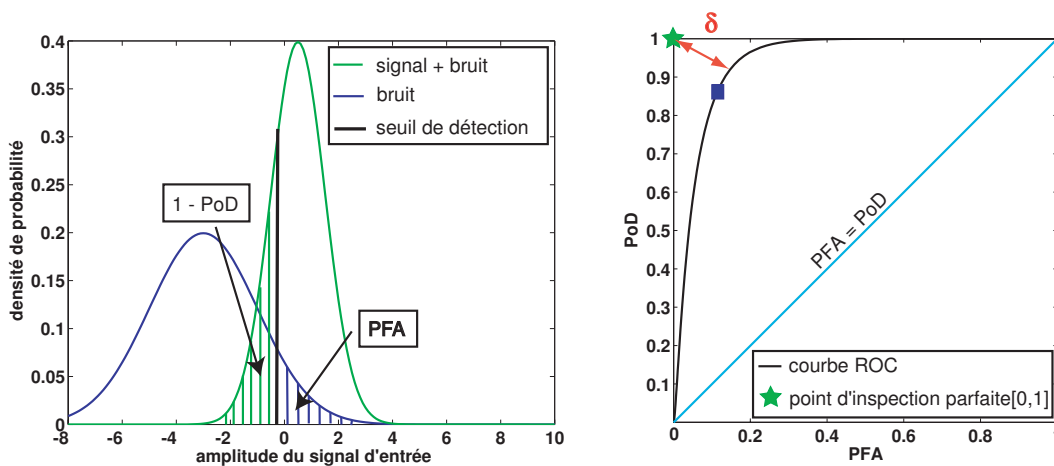
FIG. 4.3 – Illustration de la PoD et de la PFA pour un seuil de détection a_s donné (gauche) et courbe ROC correspondante (droite).
