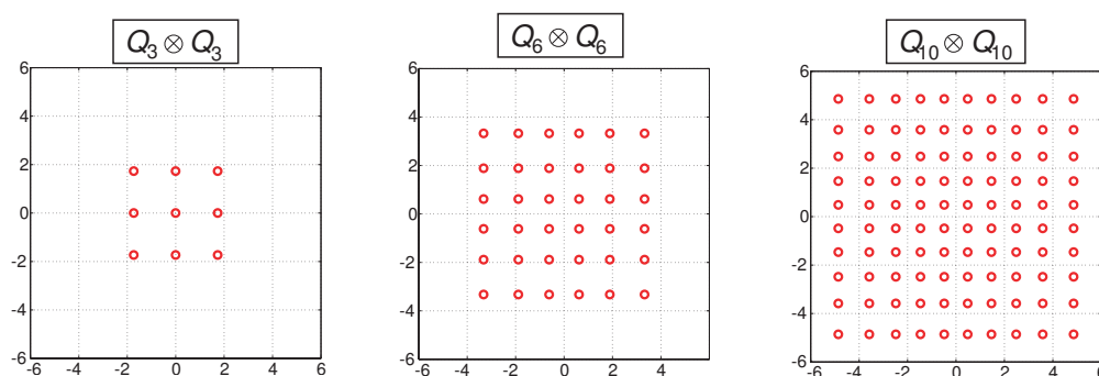
FIG. 1.3 – Exemples de quadrature de Gauss pour m = 2 et n \in \{3, 6, 10\} .
