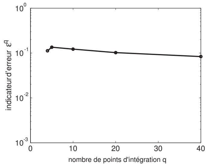
FIG. 2.25 – Exemple 2 : convergence de l'erreur \varepsilon^q en fonction de q .
