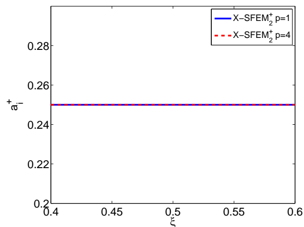
FIG. 3.14 – Exemple de référence : surfaces de réponse d'un degré de liberté enrichi obtenues avec X\text{-SFEM}_2^+ pour différents ordres de chaos polynomial p ; maillage 2 .
