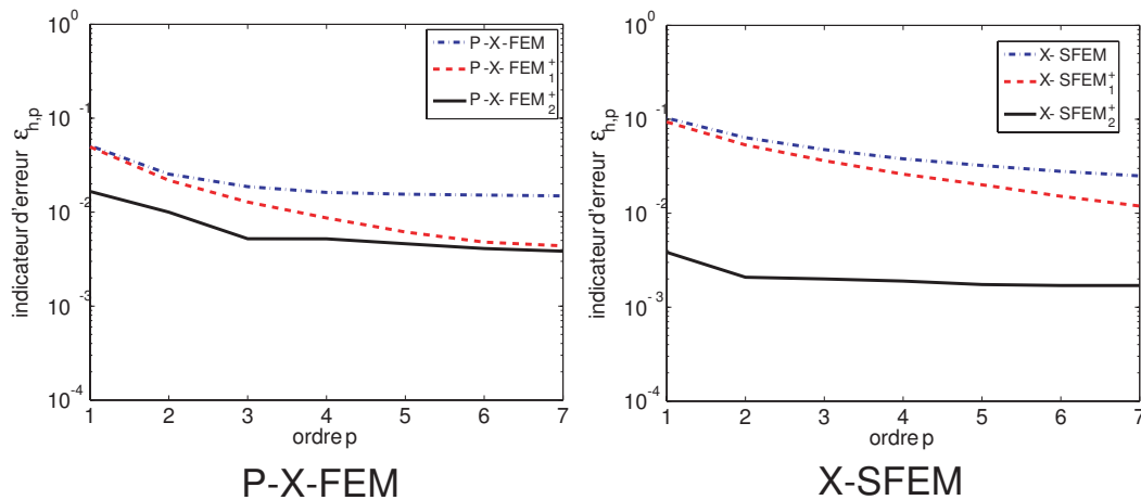
FIG. 3.26 – Exemple 1 : convergence de l'erreur \varepsilon_{h,p} en fonction de p pour les différentes solutions P-X-FEM et X-SFEM ( h = 0.06 ).
