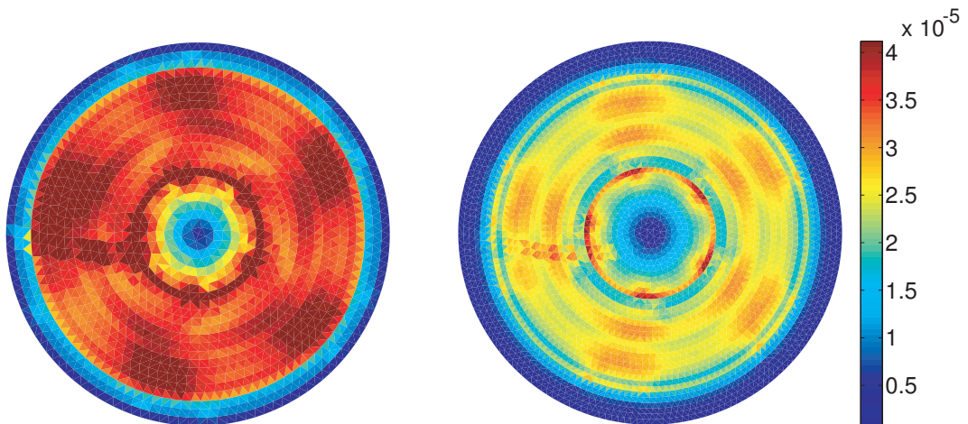
FIG. 3.25 – Exemple 1 : erreurs locales \varepsilon_{h,p}^K obtenues avec X-SFEM _2^+ pour p = 3 et h = 0.09 (gauche) et h = 0.06 (droite).
