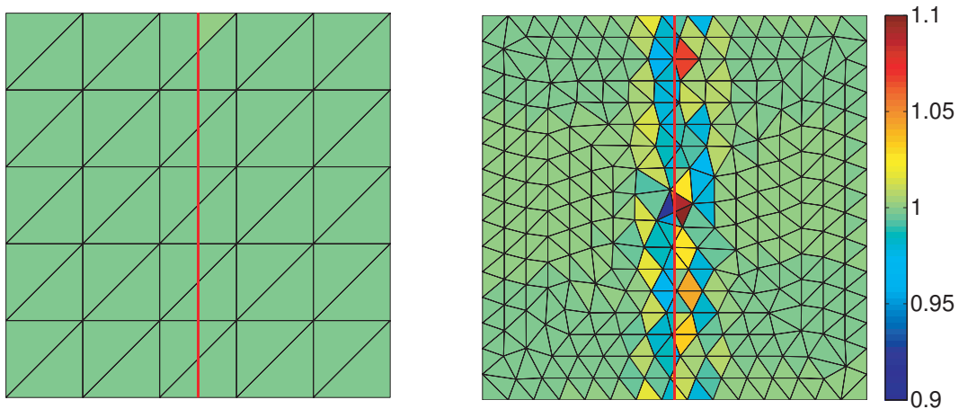
FIG. 3.10 – Exemple de référence : champs de contraintes \sigma_{xx} pour \xi = 0.5 calculés avec X-SFEM 1 + ; maillage 1 (gauche), maillage 2 (droite).
