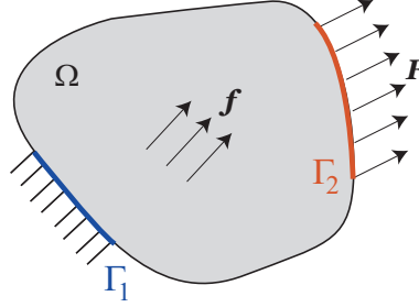
FIG. 1.2 – Problème modèle en élasticité linéaire.
