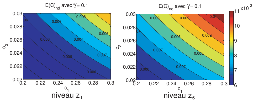
FIG. 4.15 – Evolution de la fonction de risque E(C)_{nd} dans le plan (c_1, c_2) pour les niveaux d'inspection z_1 = +2m et z_6 = -1m ; c_1 \in [0.2, 0.3] et c_2 \in [0.02, 0.03] .
