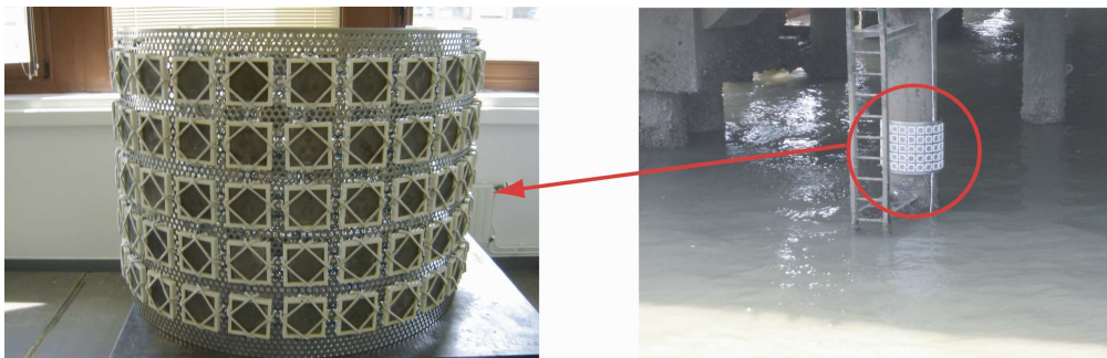
FIG. C.4 – Dispositif expérimental : support des échantillons pour le site de Saint-Nazaire.
