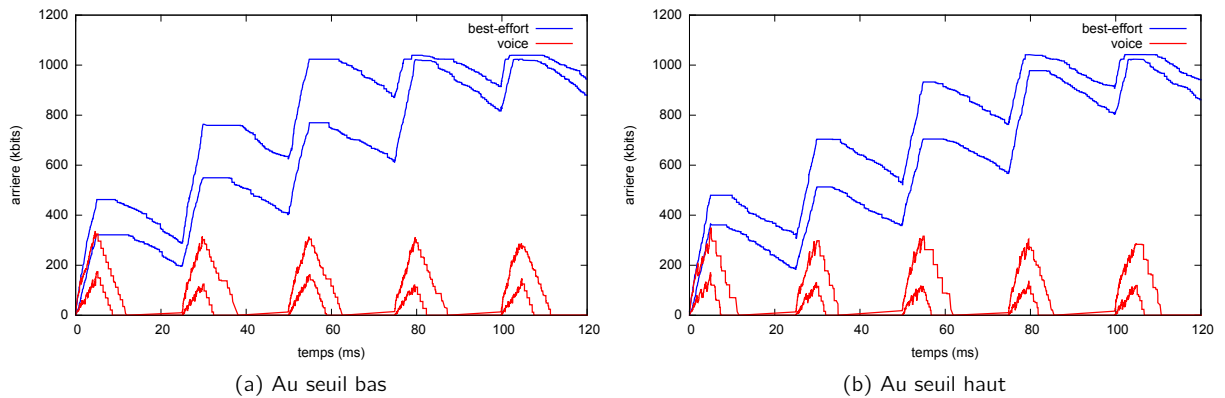
Figure 3.45 – Évolution de l'arrière de traitement lorsque le flux voice est agrégé ( e500v_{e50} )
