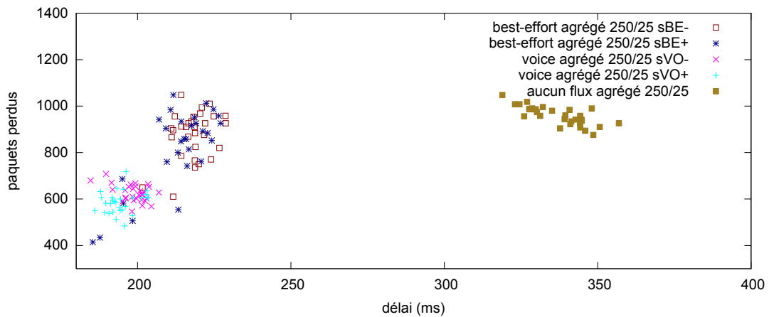
Figure 3.69 – Délai maximum, flux best-effort , e_{250v_{e25}} (avec pertes)
