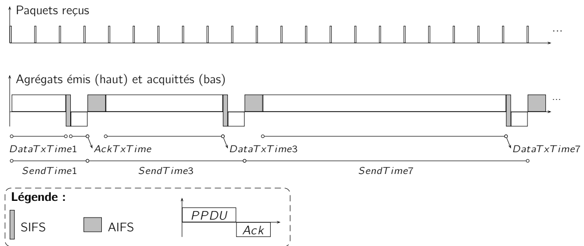
Figure 2.20 – Chronogramme entre entrée et sortie de la couche MAC de 802.11n lorsque l'agrégation est active
