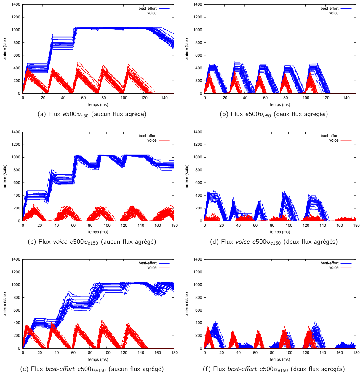
Figure 3.32 – Évolution de l'arrière lors de l'augmentation de l'inter-arrivée des paquets (aucun puis deux flux agrégés)
