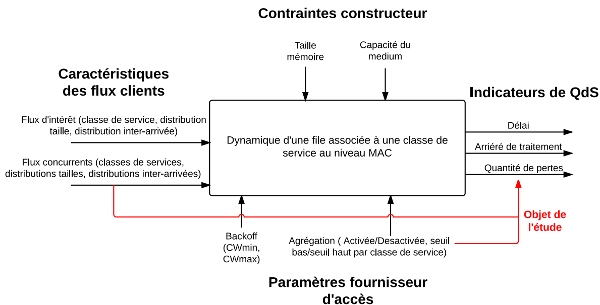
Figure 3.1 – Représentation du système sous forme de boîte noire et positionnement des différentes contraintes, indicateurs et paramètres du système
