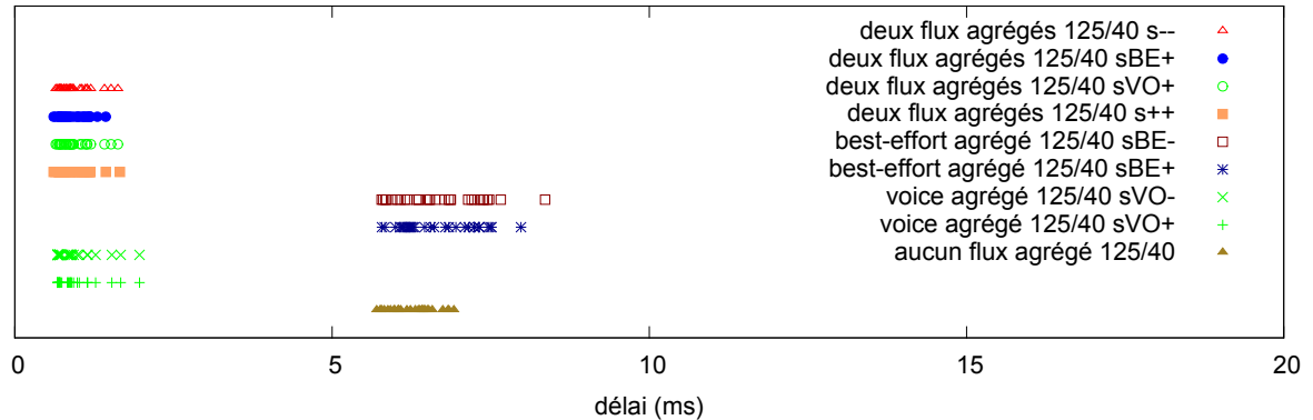
Figure 3.68 – Délai maximal pour le flux voice ( e_{125v_{e40}} )
