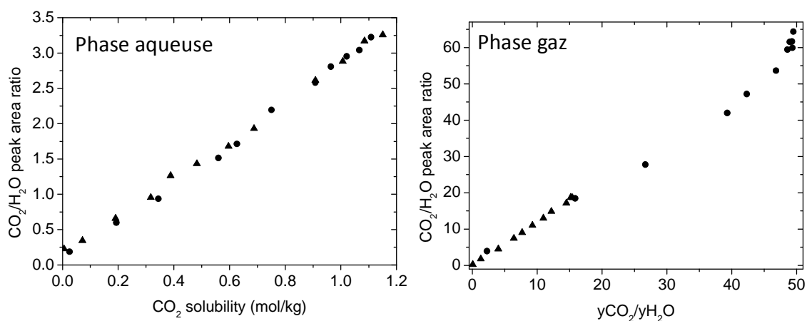
Figure 10 : Rapport des pics d'intensité Raman de CO_2 et H_2O reportés en fonction de la solubilité du CO_2 dans la phase aqueuse et du rapport molaire des phases CO_2 et H_2O dans la phase gaz. Les données théoriques sont issues du modèle de Duan et al. 2003. Expériences à 150°C (triangles) et 100°C (cercles).
