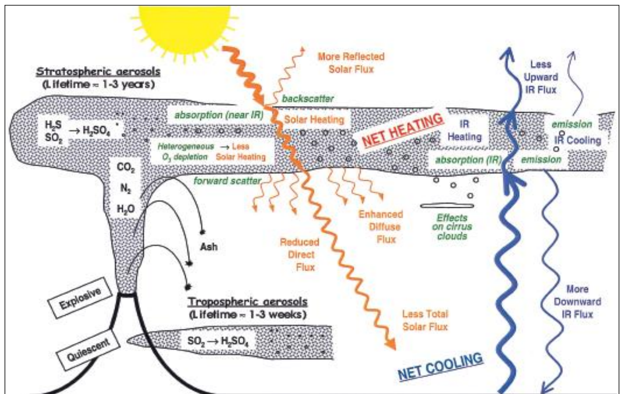
Fig.90 : Conséquences d'une éruption volcanique sur le climat.
