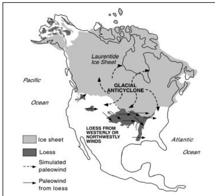
Fig.101 : Reconstitution des paléo-vents ayant soufflé sur les grandes plaines de l'Amérique du Nord en fonction du dépôt des loëss pendant le DMG Source : MUHS D.R. et BETTIS III E.A., (2000)
