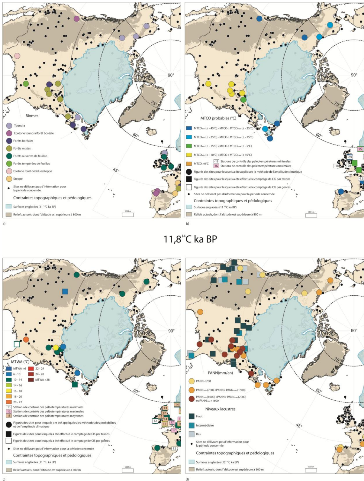
Fig.22 : Caractéristiques bioclimatiques de l'Amérique du Nord (11 800 14C BP)
