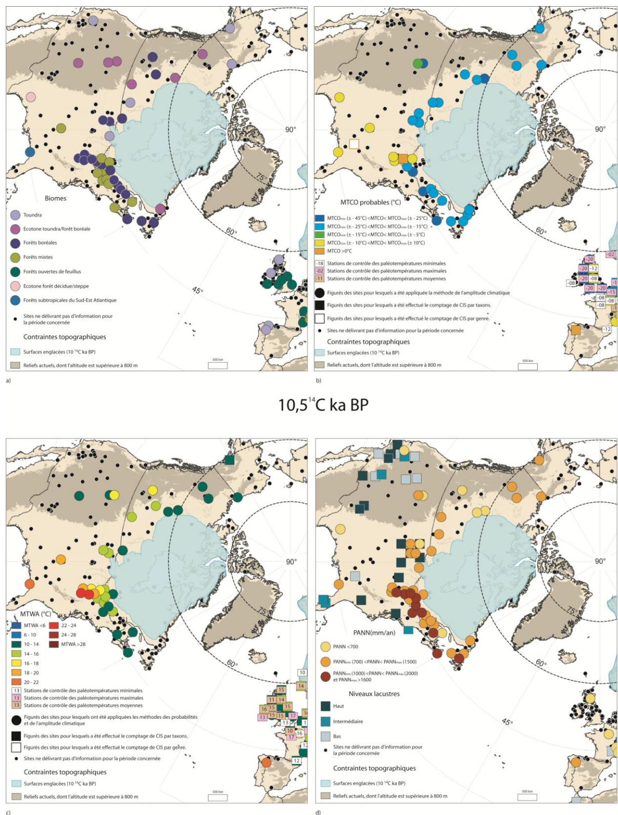
Fig. 29 : Caractéristiques bioclimatiques de l'Amérique du Nord (10 500 14 C BP)
