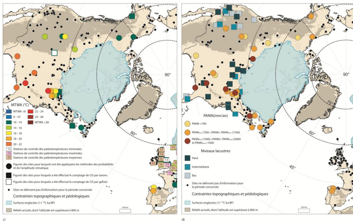
Fig.23 : Caractéristiques bioclimatiques de l'Amérique du Nord (11 500 14 C BP)
