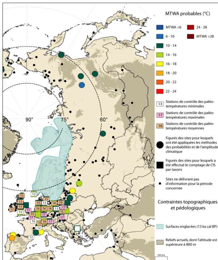
Fig.53 : Quantifications des MTWA proposées par l'équipe MPDB pour la période 11 300 (± 200) 14 C BP
