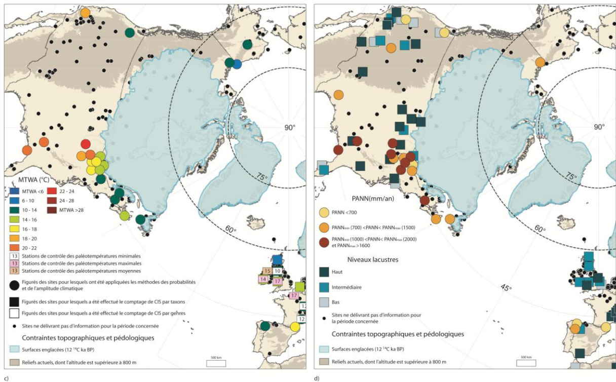
Fig.21 : Caractéristiques bioclimatiques de l'Amérique du Nord (12 000 14 C BP)
