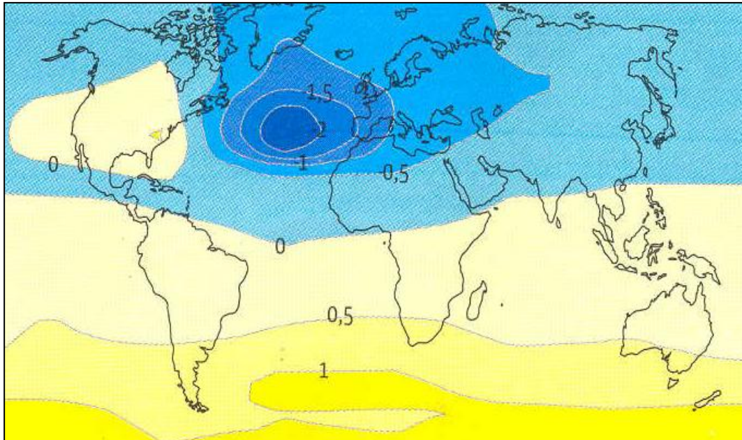
Fig.75 : Impact climatique global d'un événement d'HEINRICH, simulé grâce à un modèle de complexité réduite.
