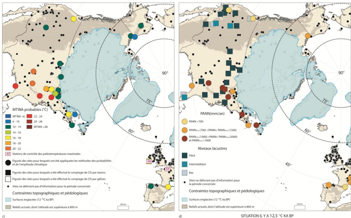
Fig.20 : Caractéristiques bioclimatiques de l'Amérique du Nord (12 300 14 C BP)
