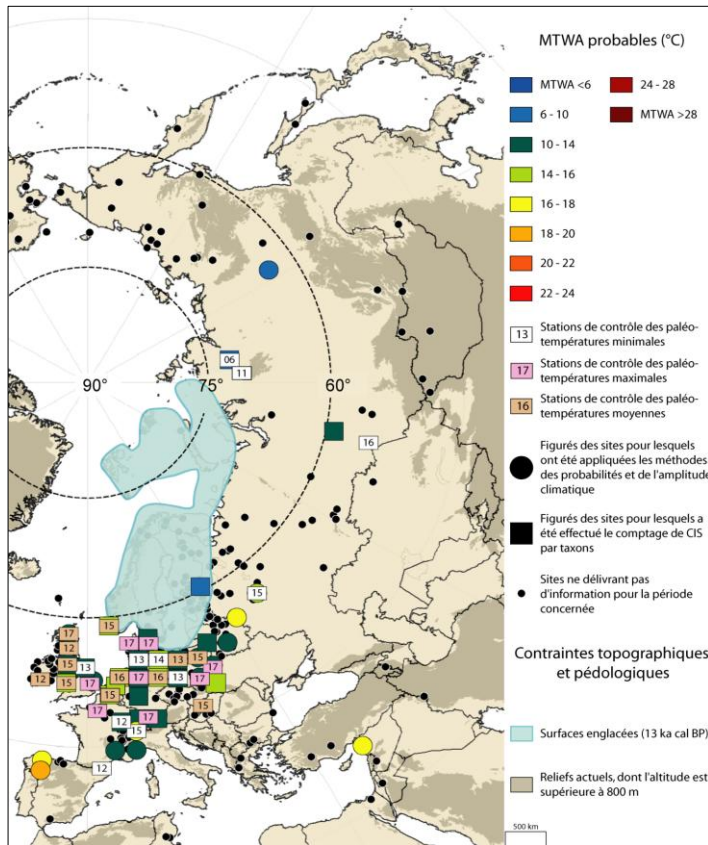
Fig.52 : Quantifications des MTWA proposées par l'équipe MPDB pour la période 11 500 (± 300) 14 C BP
