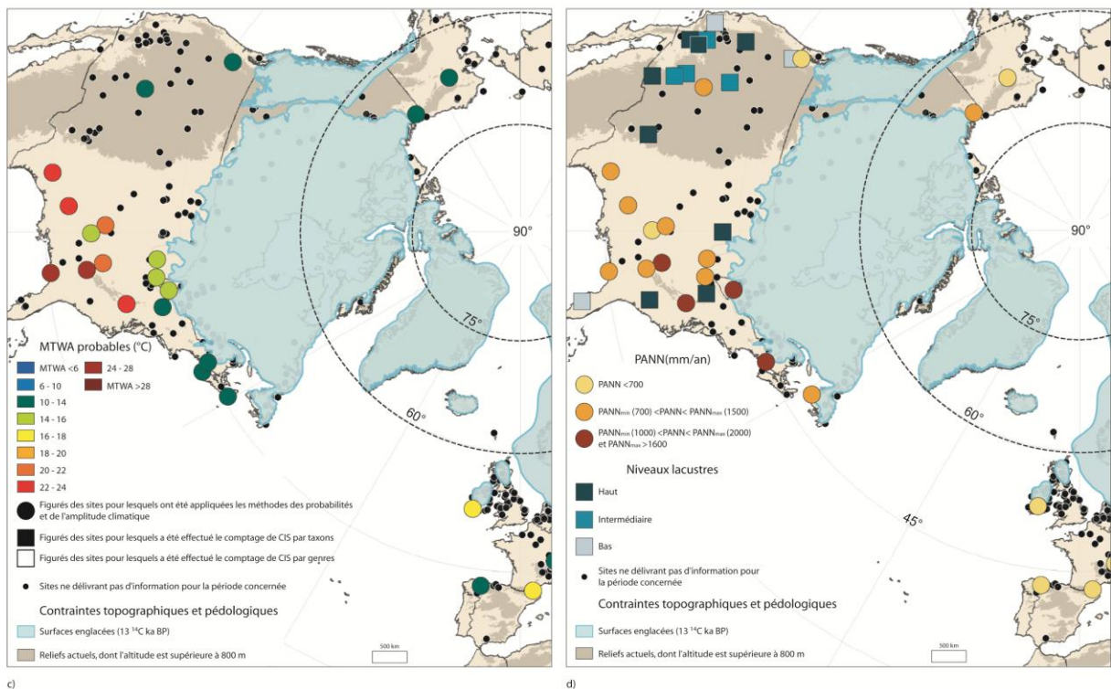
Fig.15 : Caractéristiques bioclimatiques de l'Amérique du Nord (13 500 14C BP)
