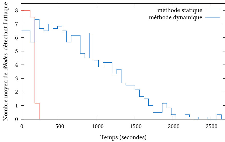
FIG. 4.13 : Détection des attaques de déni de service
