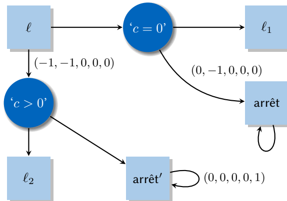
FIG. 7.4 : Module d'encodage de l'instruction 0 -test sous forme de jeu : « si c = 0 alors aller   l' tiquette \ell_1 , sinon d cr menter c et aller   l' tiquette \ell_2 ». Les  tats sous forme de carr s appartiennent au joueur 0, les cercles repr sentent les  tats du joueur 1. Il est convenu qu'en l'absence d'indication de poids, les ar tes comportent les poids (0, 0, 0, 0, 0) .
