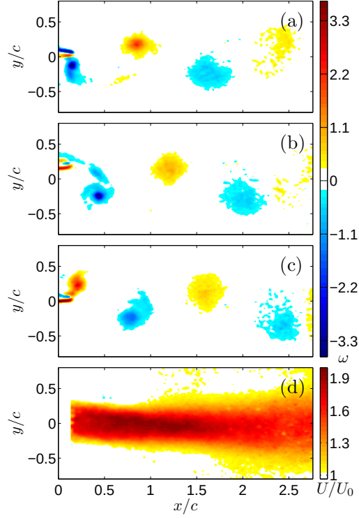
FIGURE 3.17 – Champ de vorticité expérimental créé par le battement de la plaque flexible pour différents phasages du battement de la plaque. Les déphasages sont (a) \pi/2 , (b) \pi et (c) 3\pi/2 . Les conditions expérimentales sont Re = 6000 pour la plaque B1, l'amplitude d'activation est de A_{LE} = 0.004 m et la fréquence est proche de la résonance \Omega/\Omega_0 \sim 1 . (d) Vitesse moyenne temporelle U générée par le mouvement de la plaque relative à l'écoulement imposé U_0 .
