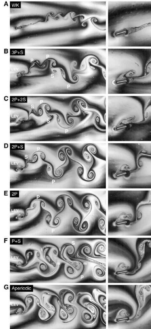
FIGURE 3.12 – (gauche) Classification des sillages derrière un cylindre, tiré de Williamson et Roshko (1988) [90]. “S” signifie un vortex isolé tandis que “P” correspond à une paire de vortex lâchée dans le sillage. (droite) Visualisations de correspondance derrière une plaque plane rigide oscillant dans un film de savon, tiré de Lentink et al. (2008) [47].
