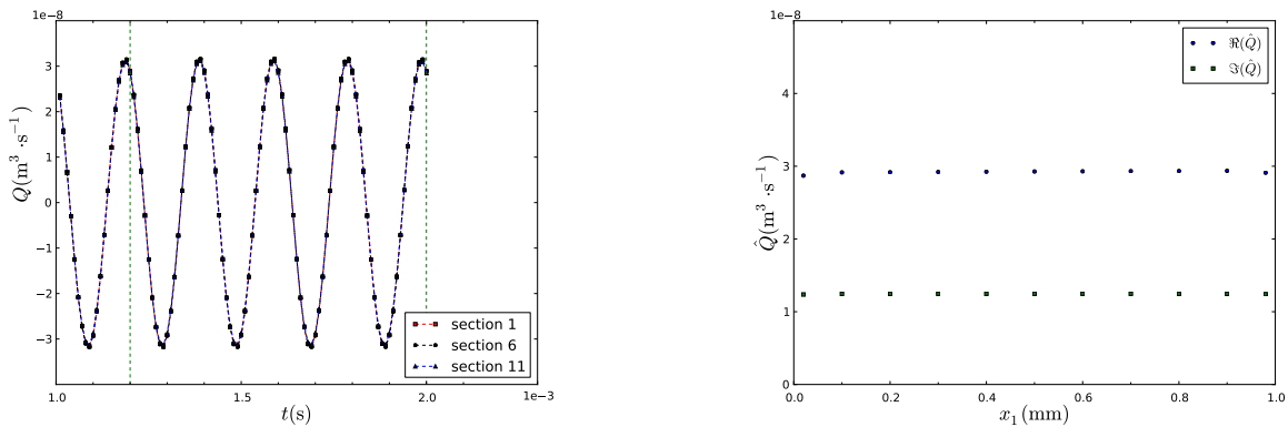
(a) Evolution temporelle du débit volumique dans trois sections
