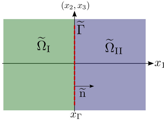
FIGURE 1.4 – Schéma de la zone de champ lointain.
