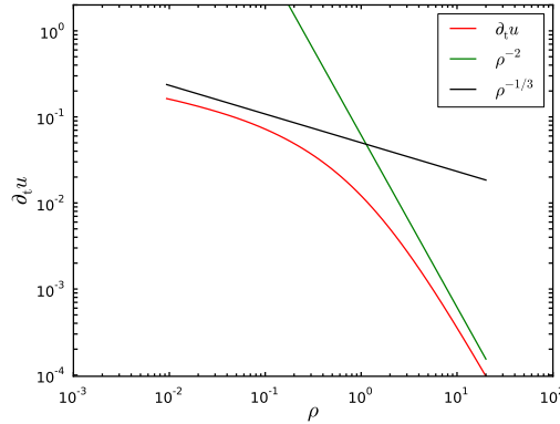
FIGURE 4.4 – Comportement asymptotique de la dérivée tangentielle de u
