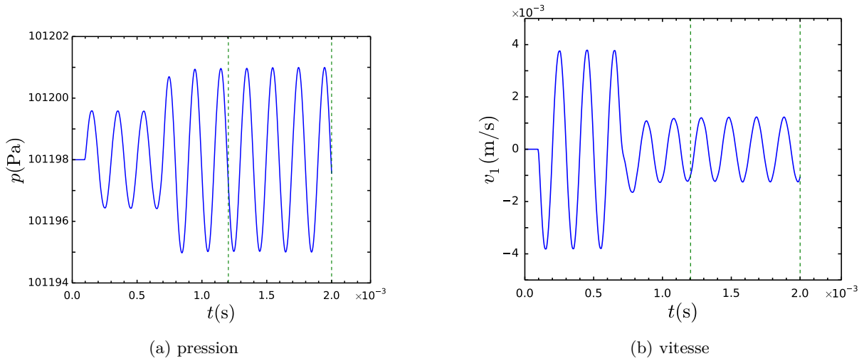
FIGURE 5.3 – Evolution temporelle de la pression et de la vitesse axiale enregistrée par le capteur numérique 5.
