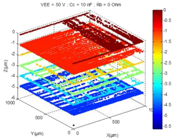
Distribution spatiale des décharges / Empilement des couches
