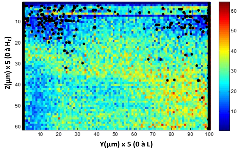
Figure 117 – Superposition de la cartographie des contacts et de la représentation en couleur des décharges ( H_c = 300 \mu m ). Echelle en X et Y : 5 \mu m / unité.
