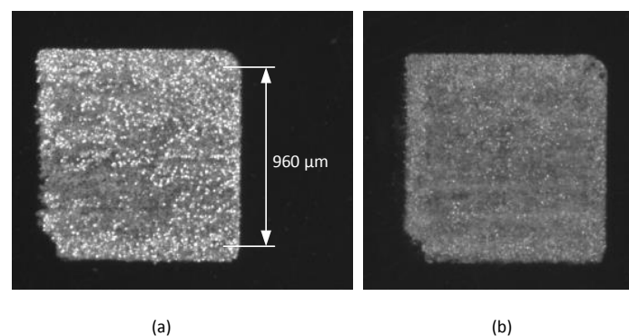
Figure 156 – Etat de surface d'une cavité usinée. (a) R_b = 0 \Omega . (b) R_b = 100 \Omega .
