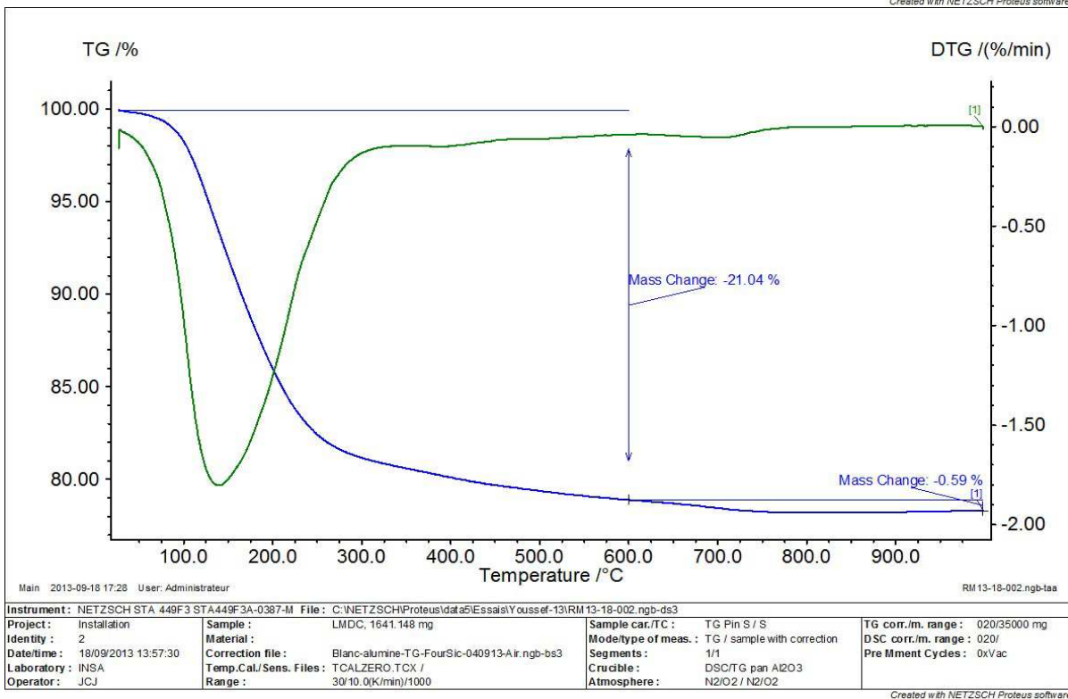
Figure 85: Analyse thermique de la pâte hydratée du liant T^L à 28 jours
