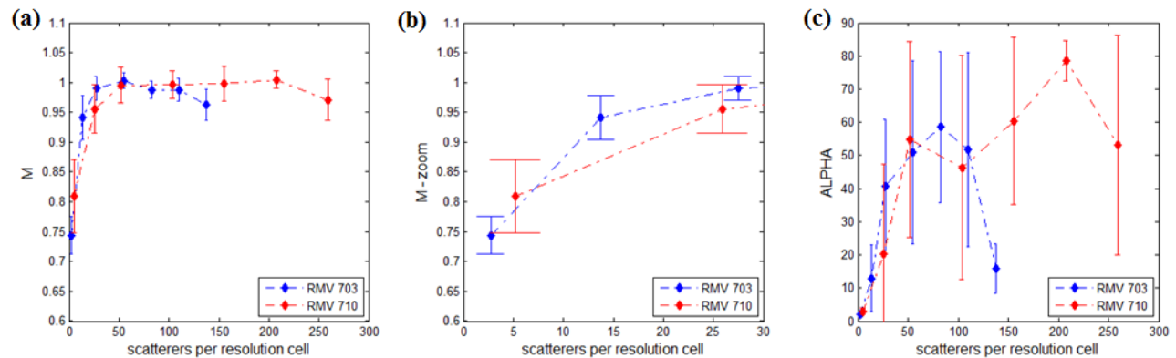
Figure 11 Paramètres de forme des deux distributions en fonction du nombre de diffuseurs par cellule de résolution (a) Paramètre m de Nakagami (b) Paramètre m de Nakagami – concentrations basses (c) Paramètre \alpha de la K-Homodyne
