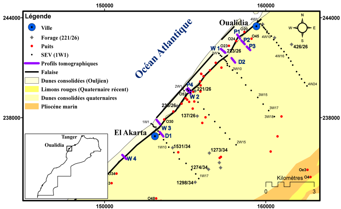
FIGURE 6.1 – Emplacement des sondages électriques verticaux (DRPE 1992) et des profils de tomographie de résistivité électrique (2012 et 2013)
