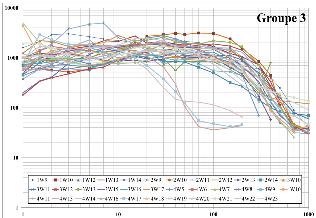
FIGURE D.3 – Les pseudosondages verticaux du groupe 3
