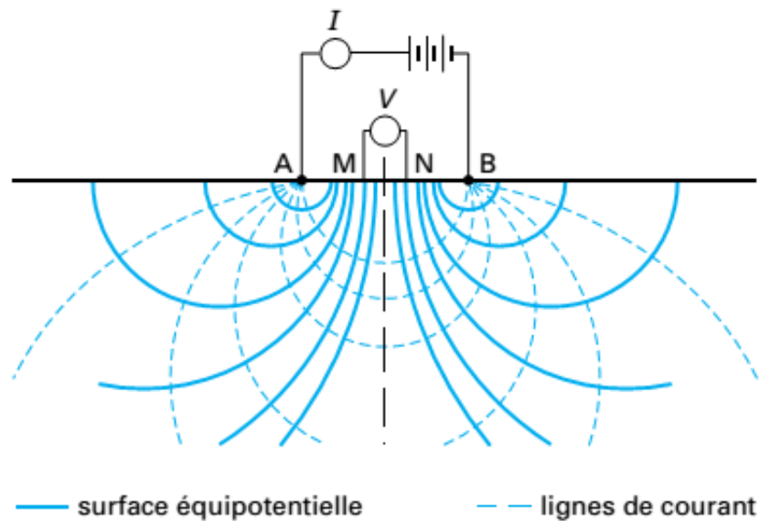
FIGURE 2.3 – Distribution du courant créé par deux électrodes dans un sol homogène et isotrope (d'après Van Nostrand et Cook, 1966)
