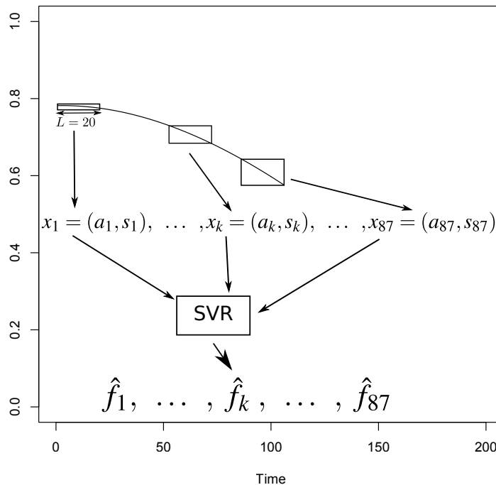
FIGURE 5.9 – Estimation du RUL d'un nouveau composant U en utilisant le modèle SVR construit au préalable : Les caractéristiques de tendance sont extraites de fenêtres coulissantes et le modèle SVR qui estime le RUL de chaque fenêtre. Dans cet exemple, L = 20 et l(u) = 106 .
