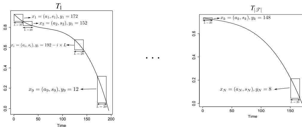
FIGURE 5.8 – Description schématique d'extraction de caractéristiques de tendance à partir des séries temporelles et leurs valeurs du RUL associées. Dans cet exemple, L = 20 , l(T_1) = 192 , et l(T_1|\mathcal{T}) = 158 .
