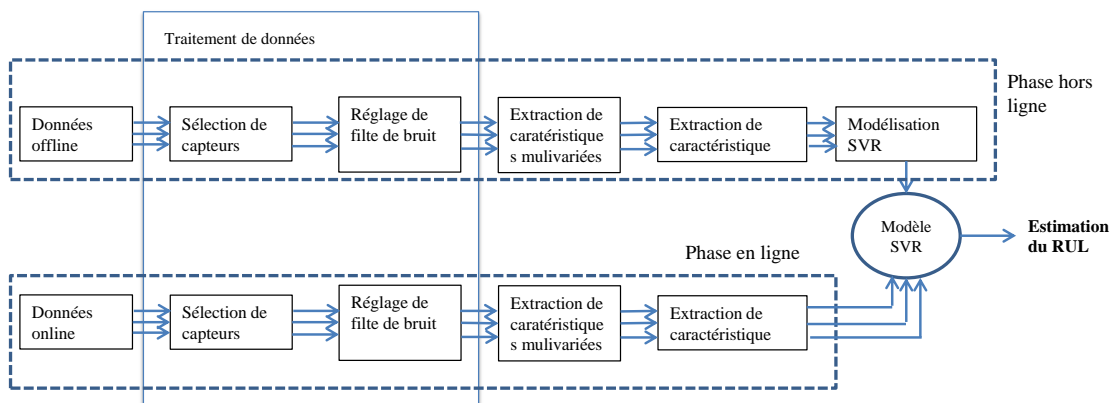
FIGURE 5.13 – L'approche développée sur des signaux multidimensionnels.
