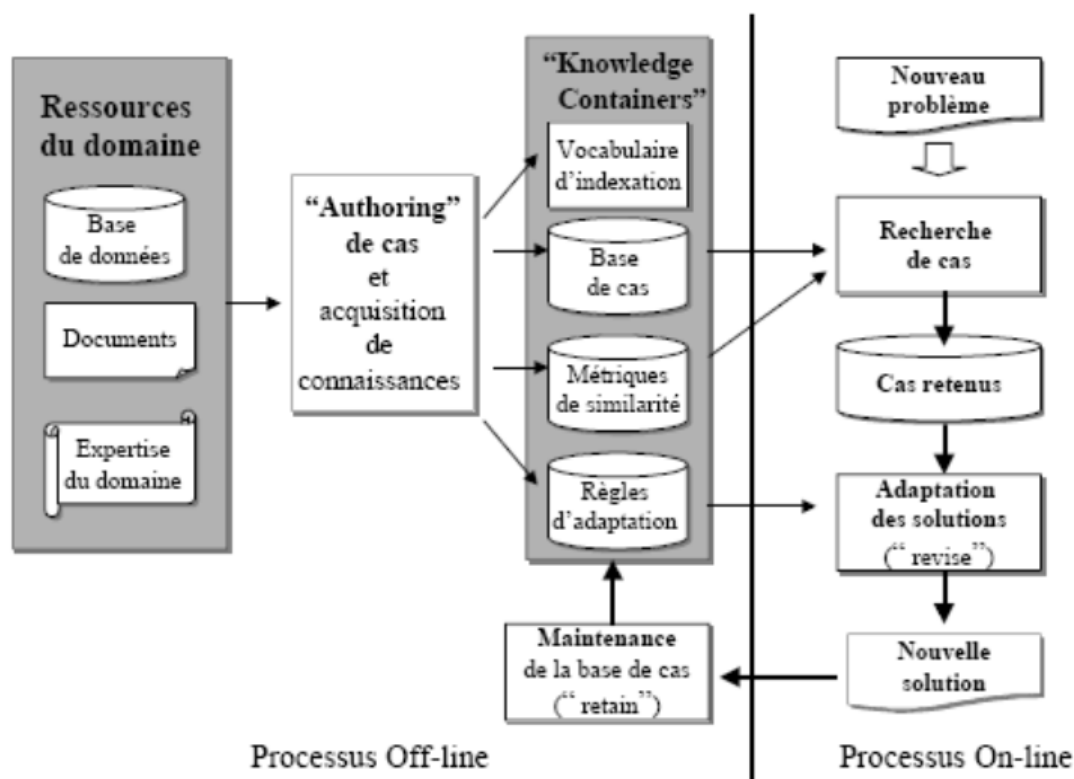
FIGURE 4.5 – Modèle générique d'un système de RàPC [Lamontagne et al., 2002].
