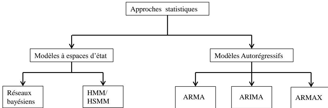
FIGURE 2.8 – La classification des approches statistiques.
