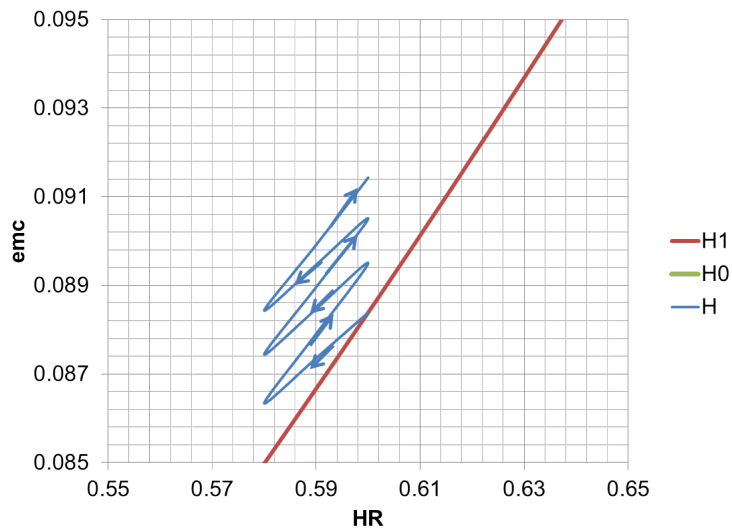
FIGURE 3.44 – Détail de l'isotherme de sorption à 20°C implémenté dans TransPore 3D (Perré 1999). On décrit ici une succession de séchage et d'humidification pour de petites amplitudes d'humidité. Le calcul de l'humidité interne diverge.
