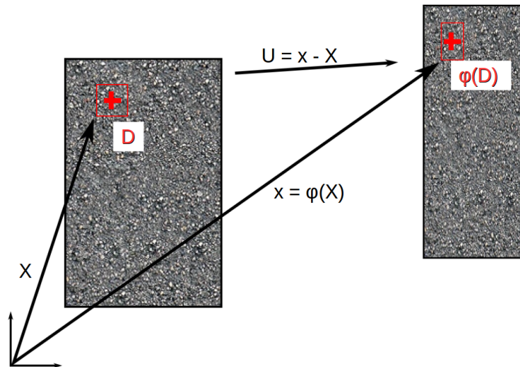
FIGURE 1.17 – Principe de la corrélacion d'images numériques.
