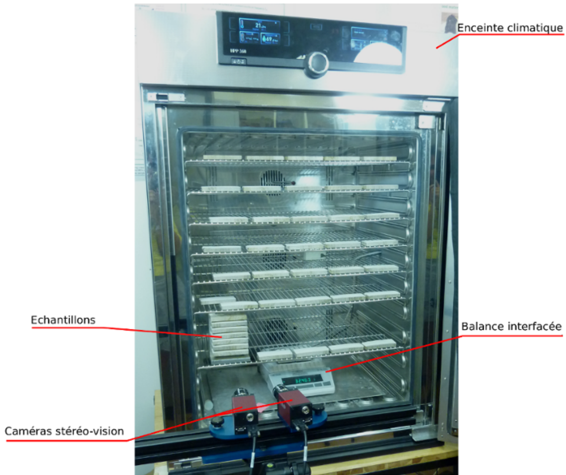
FIGURE 2.22 – Montage expérimental.
