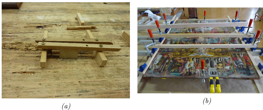
FIGURE 1.32 – Travail de remise à niveau de la courbure locale (a) (travail effectué par Brita New à la National Gallery de Londres) et globale (b) (travail effectué par Daniel Jaunard et Gilles Tournillon au musée Fabre de Montpellier).
