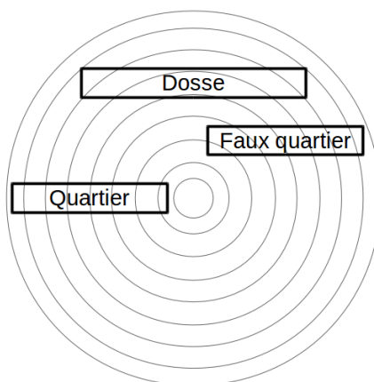
FIGURE 1.24 – Schéma de débits classiques dans une grume.
