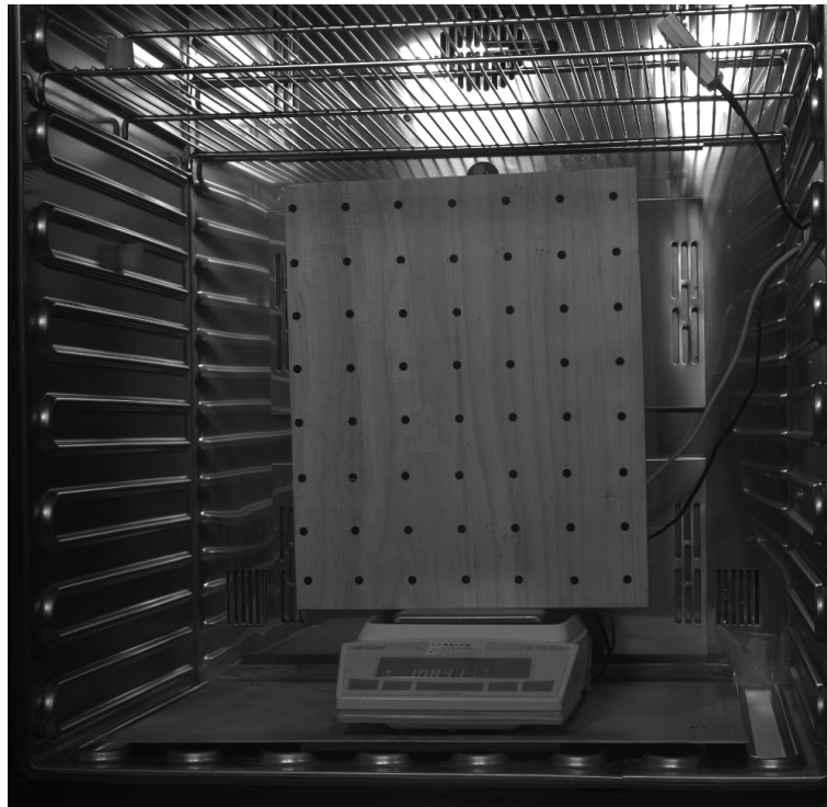
FIGURE 3.3 – Photo du panneau dans l'enceinte climatique sur la balance interfacée.
