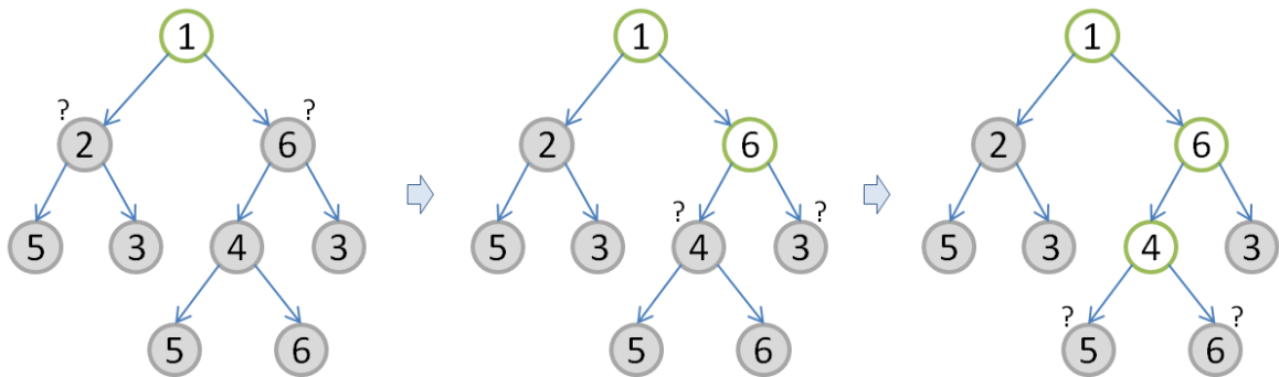
Figure 50. Parcours de l'arbre pour la reconnaissance automatique de tâches chirurgicales
