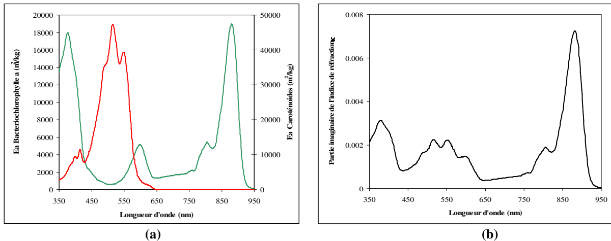
Figure II.28 : Reconstitution de la partie imaginaire de l'indice de réfraction \kappa_{\lambda} (b) de Rhodospirillum rubrum par convolution (ég. II.6.4) à partir des coefficients d'absorption in vivo des pigments purs (a). Les teneurs massiques utilisées sont 1,75% de bactériochlorophylle a ( — ) et 0,35% de caroténoïdes (spirilloxanthine et rhodovibrine — ).
