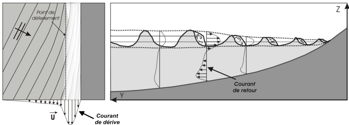
FIGURE 1.7 – Illustration des courants de dérive (gauche) et de retour (droite) induits par les vagues en zone côtière. Source : Castelle (2004).
