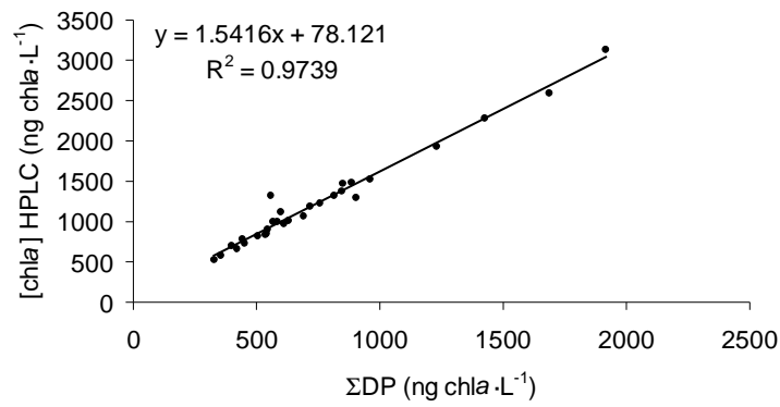
Figure 6 : Linear regression between HPLC chl a concentration vs the sum of diagnostic pigments ΣDP (peri+fuco+19BF+19HF+allo+zea+chl b ) for the « oceanic » area . Régression linéaire obtenue entre les concentrations en chl a (HPLC) et la somme de biomarqueurs ΣDP (peri+fuco+19BF+19HF+allo+zea+chl b ) pour le réseau « océanique ».
