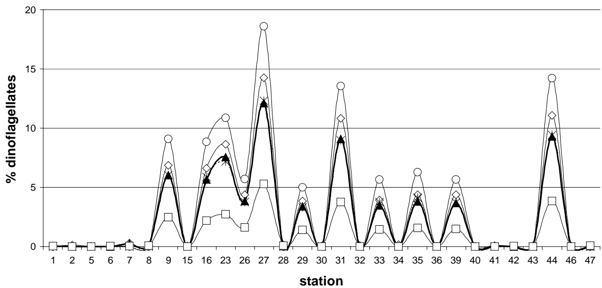
Figure 8 : Pourcentage of Cryptophytes and Dinoflagellates in the « oceanic » area stations calculated by : star : DP method ; circle : Multiples Regressions ; diamond : Chemtax A ; triangle : Chemtax B ; square : Chemtax C . Pourcentage de cryptophycées et dinoflagellés sur le réseau « océanique » selon les méthodes : étoile : DP method ; cercle : Multiples Regressions ; losange : Chemtax A ; triangle : Chemtax B ; carré : Chemtax C .
