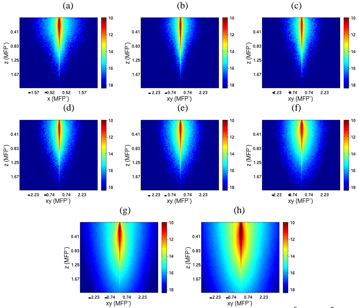
Figure IV.26: Coupe transversale de la PPSDF entre les valeurs d'intensité 1.5 \cdot 10^{-8} et 4.5 \cdot 10^{-8} (u.a.) [ \sim \exp(-18) et \exp(-10) (u.a.) sur la figure]. Coupe transversale horizontale pour la polarisation (a) linéaire, coupe transversale diagonale pour la polarisation (b) elliptique ( \epsilon=0\pi ), (c) elliptique ( \epsilon=0.05\pi ), (d) elliptique ( \epsilon=0.1\pi ), (e) elliptique ( \epsilon=0.15\pi ), (f) circulaire ( \epsilon=0.25\pi ), (g) dépolarisé et (h) sans polarisation. Aucune inclusion n'est présente dans le milieu homogène et semi-infini.
