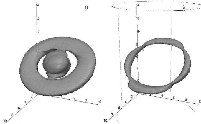
Figure IV.20: Reconstruction des paramètres optiques en 3D. Isosurface du coefficient de transport (gauche) et de l'albedo (droite). (Soloviev et al. 2012)
