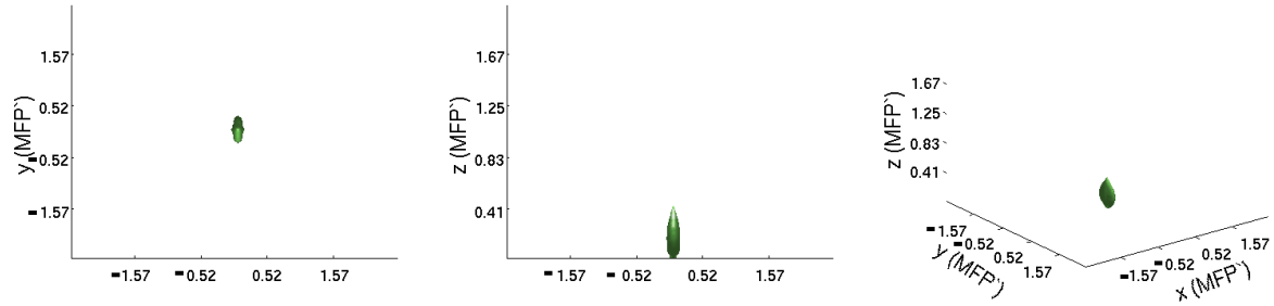
Figure IV.8: Représentation du volume sondé par le flux de photons ayant une intensité de la valeur 5 \cdot 10^{-6} (u.a.). La polarisation maintenue est linéaire et la vue sur le volume s'effectue par l'intérieur du milieu sondé comme ainsi : (a) en direction de l'axe z, (b) latéralement en direction de l'axe y, (c) diagonalement.
