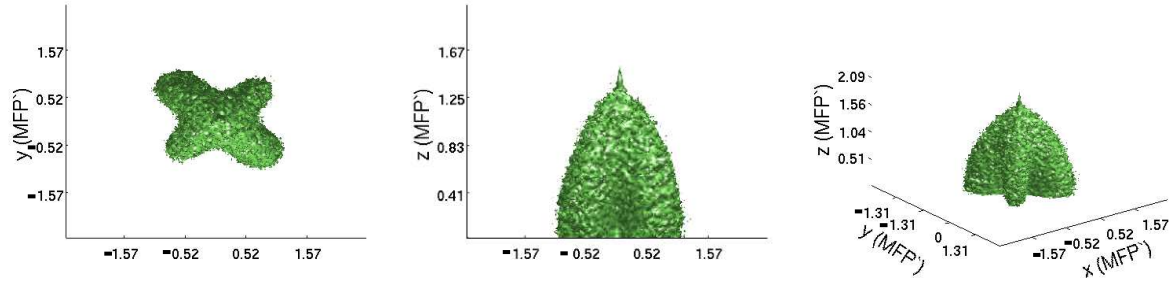
Figure IV.31: Représentation du volume de la PPSDF pour la polarisation maintenue elliptique ( \epsilon=0.15 \pi ) avec une vue (a) dans la direction de l'axe z, (b) latérale dans la direction de l'axe y et (c) diagonale incliné. Les figures montrent une représentation vue depuis le milieu.
