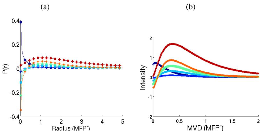
Figure III.25: Soustraction du canal contre-polarisé du canal co-polarisé pour (a) l'intensité rétrodiffusée et pour (b) la profondeur moyenne sondée. Les polarisations représentées sont: linéaire ( \epsilon=0 ), elliptique ( \epsilon=0.05\pi ), elliptique ( \epsilon=0.1\pi ), elliptique ( \epsilon=0.15\pi ), circulaire ( \epsilon=0.25\pi ) et dépolarisé. L'ellipticité est exprimée avec \epsilon . Le milieu choisi a les paramètres optiques suivants : \mu_a=0.5 \text{ cm}^{-1} , \mu_s=50 \text{ cm}^{-1} et g=0.8 .
