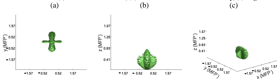
Figure IV.6: Représentation du volume sondé par le flux de photons ayant une intensité de la valeur 5*10^{-7} (u.a.). La polarisation maintenue est linéaire et la vue sur le volume s'effectue par l'intérieur du milieu sondé comme ainsi : (a) en direction de l'axe z, (b) latéralement en direction de l'axe y, (c) diagonalement.
