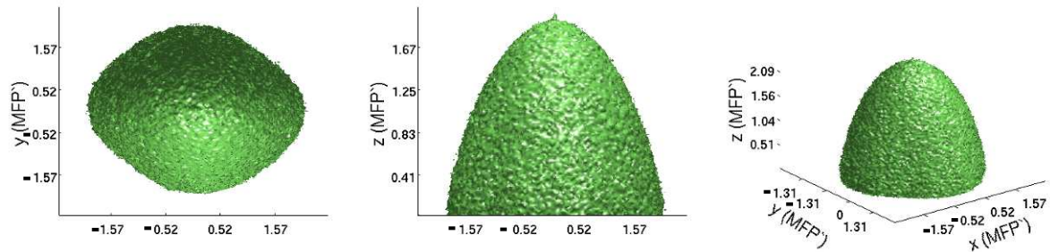
Figure IV.33: Représentation du volume de la PPSDF pour les photons multiplément diffusée avec une vue (a) dans la direction de l'axe z, (b) latérale dans la direction de l'axe y et (c) diagonale incliné. Les figures montrent une représentation vue depuis le milieu.
