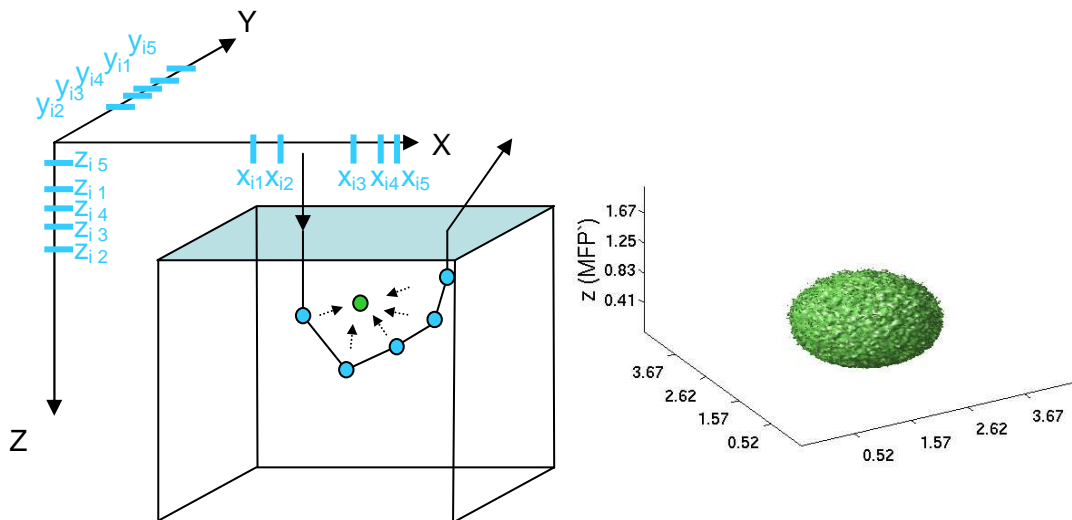
Figure II.12 : (a) Schéma illustrant la sauvegarde du volume sondé par un photon rétrodiffusé. Exemple de résultat issu d'une simulation Monte Carlo pour le volume sondé par des photons non polarisés (b).
