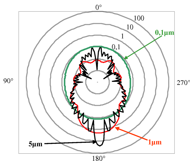
Figure I.7: Indicatrices de diffusion pour des sphères de diamètres 0.1 µm (en vert), 1µm (en rouge) et 5µm (en noir). L'indice de réfraction du milieu environnant est 1, celui des sphères est 1.4, le faisceau à une incidence de 0°, et la longueur d'onde est de 0.633 µm.
