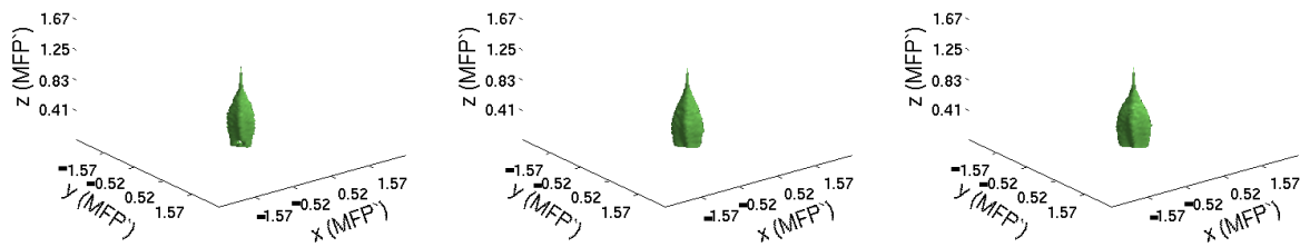
Figure IV.37: Représentation de l'extension en trois dimensions de la PPSDF pour la polarisation elliptique ( \epsilon=0.15\pi ) et une inclusion aux profondeurs: (a) 0.06 MFP' (60 \mu\text{m} ), (b) 0.25 MFP' (240 \mu\text{m} ) et (c) 0.42 MFP' (400 \mu\text{m} ).
