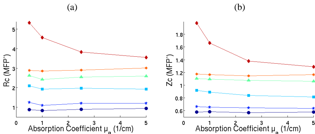
Figure III.13: Comportement de du descripteur (a) radial à 90% de la surface et (b) de la profondeur moyenne à 10% du maximum pour une variation du coefficient d'absorption. Les polarisations représentées sont: linéaire ( \epsilon=0 ), elliptique ( \epsilon=0.05\pi ), elliptique ( \epsilon=0.1\pi ), elliptique ( \epsilon=0.15\pi ), circulaire ( \epsilon=0.25\pi ) et dépolarisé. L'ellipticité est exprimée avec \epsilon .
