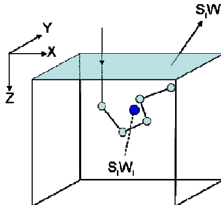
Figure IV.1: Schéma de principe pour obtenir la position moyenne du trajet d'un photon rétrodiffusé. La quantité S_i W_i (vecteur de Stokes final pondéré) rétrodiffusée est sauvegardée au barycentre du trajet, représenté en bleu foncé.
