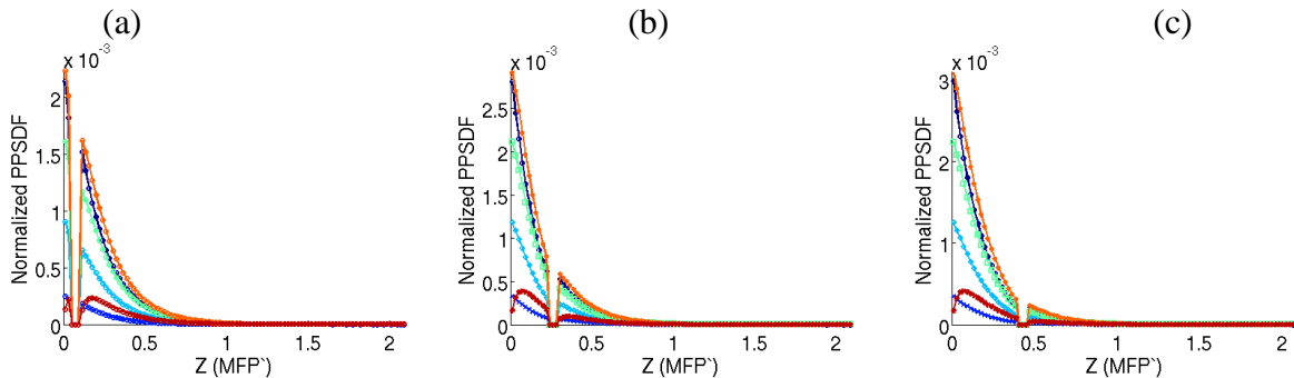
Figure IV.36: Profil de la PPSDF sous la source. L'influence de l'absorption est clairement visible. Code couleur : bleu foncé – linéaire, bleu claire – elliptique \epsilon=0.1\pi , turquoise – elliptique \epsilon=0.2\pi , vert claire – elliptique \epsilon=0.3\pi , orange – circulaire, rouge – multiple diffusée.
