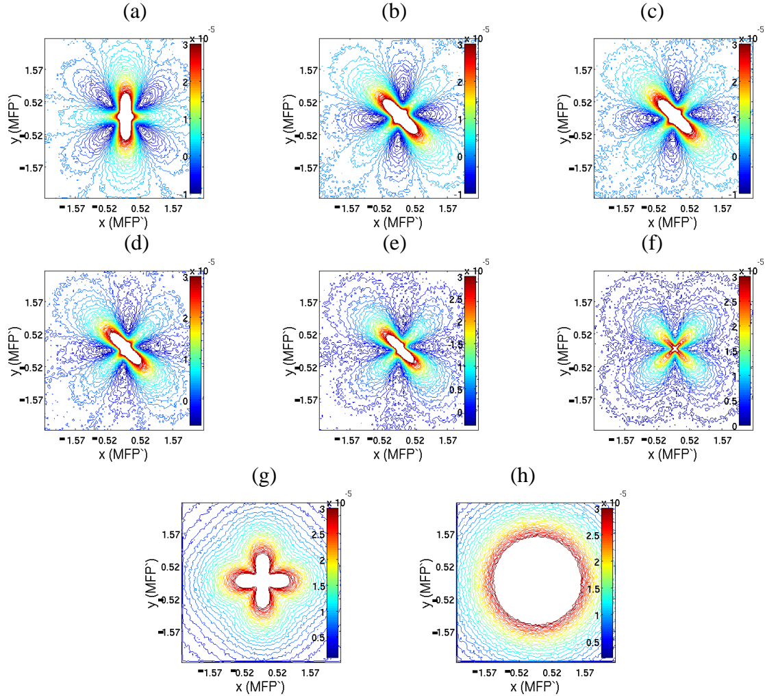
Figure IV.1: Intensités rétrodiffusées normalisées avec les polarisations maintenues : (a) linéaire horizontal, (b) linéaire 45^\circ \epsilon=0\pi , (c) elliptique \epsilon=0.05\pi , (d) elliptique \epsilon=0.1\pi , (e) elliptique \epsilon=0.15\pi , (f) circulaire \epsilon=0.25\pi , (g) multiplement diffusés (polarisation perdu) et (h) sans polarisation. Les soustractions des intensités polarisées sont limitées sur une échelle de valeurs entre -1*10^{-5} et 3*10^{-5} (u.a.).
