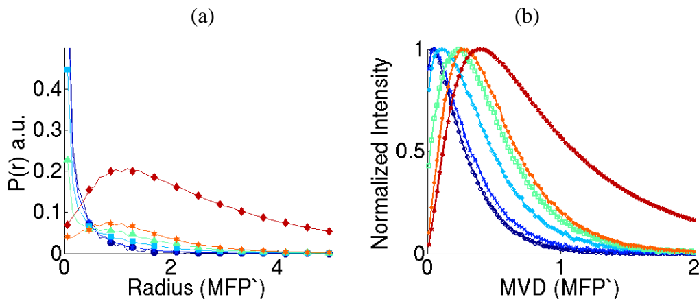
Figure III.8: (a) Exemple de l'intensité rétrodiffusée radiale. (b) Exemple de la profondeur moyenne visitée (mean visitation depth MVD). L'échelle est celle du libre transport moyen réduit ( MFP'=[\mu_a+(1-g)\mu_s]^{-1} ). Les polarisations représentés sont: linéaire ( \epsilon=0 ), elliptique ( \epsilon=0.05\pi ), elliptique ( \epsilon=0.1\pi ), elliptique ( \epsilon=0.15\pi ), circulaire ( \epsilon=0.25\pi ) et dépolarisé. L'ellipticité est exprimé avec \epsilon . Le milieu exemplaire a les paramètres optiques suivants : \mu_a=0.5 \text{ cm}^{-1} , \mu_s=100 \text{ cm}^{-1} et g=0.8 .
