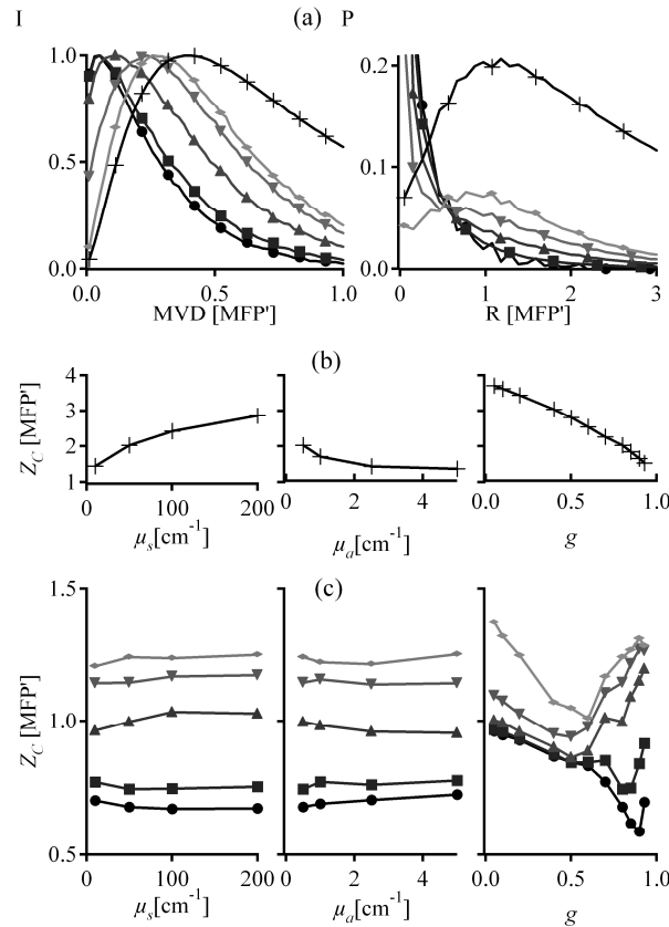
Figure III.20: (a) Montre à gauche la profondeur moyenne sondée et à droite l'intensité rétrodiffusée par les polarisations : linéaire (points), elliptique \epsilon=0.05\pi (carrés), elliptique \epsilon=0.1\pi (triangles), elliptique \epsilon=0.15\pi (triangles pointés vers le bas), circulaire (traits horizontaux) et les photons ayant perdu leur polarisation initiale (croix). (b) Evolution de Z_c de la lumière dépolarisée en fonction de \mu_a , \mu_s et g . (c) Evolution de Z_c pour différentes polarisations [comme pour (a)] en fonction de \mu_a , \mu_s et g .
