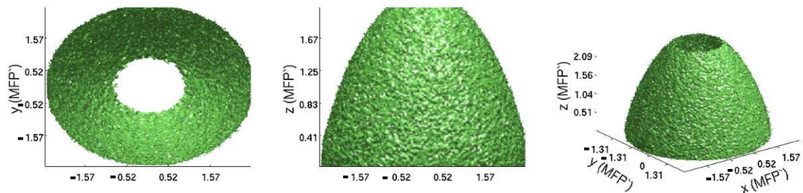
Figure IV.34: Représentation du volume de la PPSDF pour les photons sans polarisation avec une vue (a) dans la direction de l'axe z, (b) latérale dans la direction de l'axe y et (c) diagonale incliné. Les figures montrent une représentation vue depuis le milieu.
