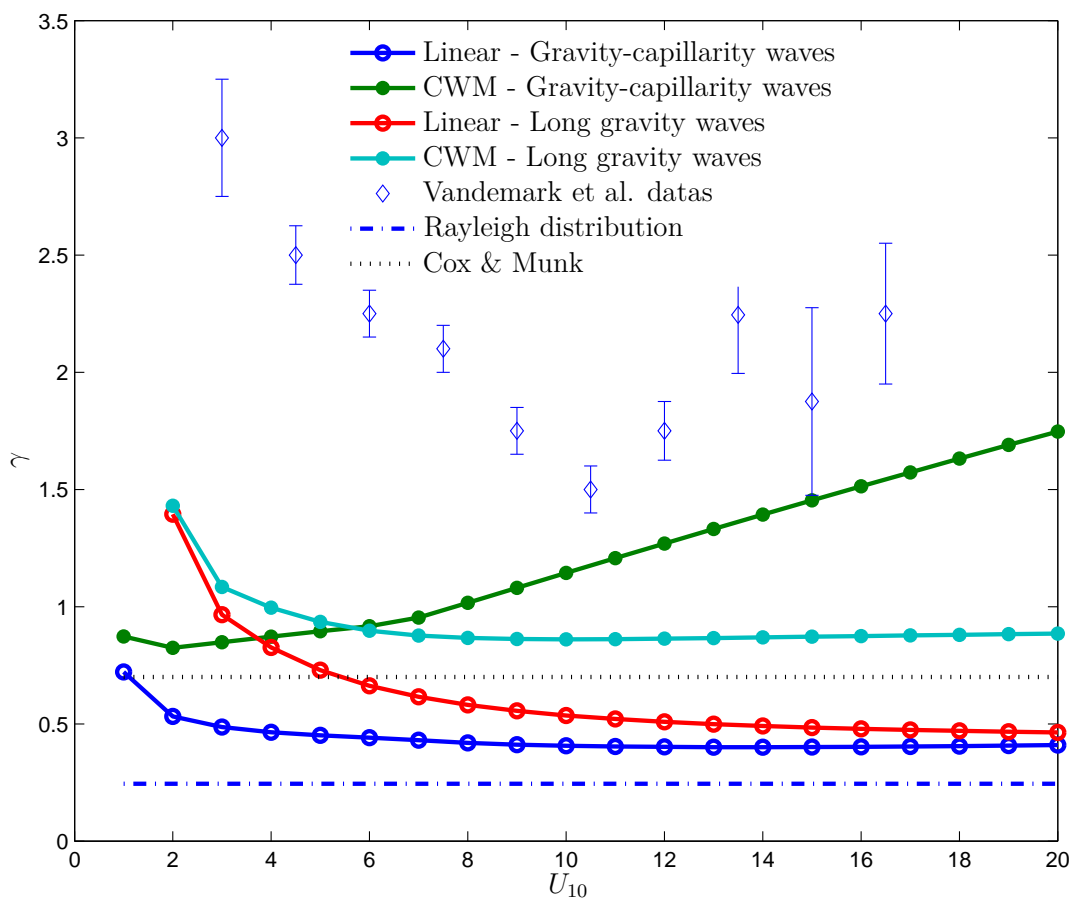
Figure 2.4 – Excès de kurtosis des pentes omnidirectionnelles comme fonction du vent.
