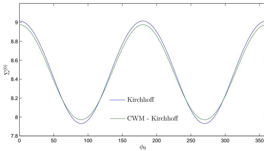
Figure 6.4 – Diagrammes azimutaux à différentes bandes, angles d'incidence et vents.
