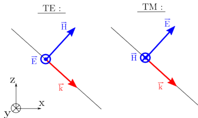
FIGURE 2.3 – Polarisation Transverse Électrique (TE) et Transverse Magnétique (TM) pour une onde incidente plane se propageant dans la direction \mathbf{k}
