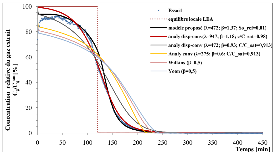
Figure IV-27: Résultats expérimentaux et de plusieurs modélisations de l'essai I/Venting
