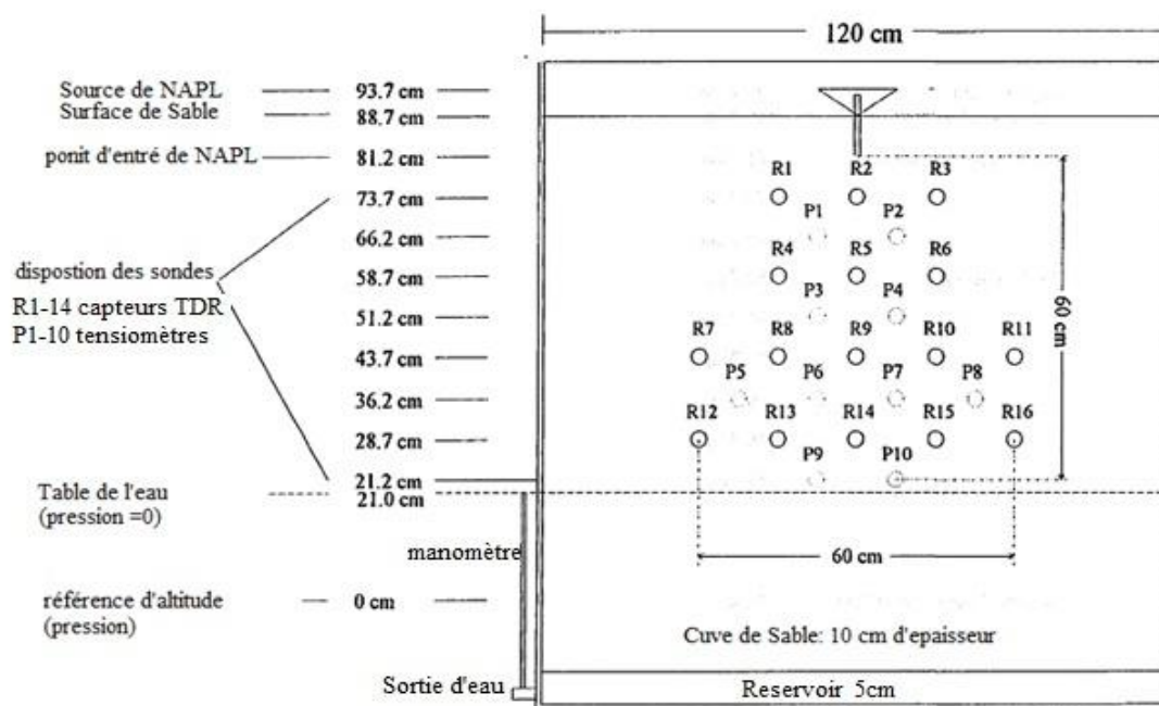
Figure II-13: Dispositif expérimental de Neumann (Neumann, 1992)
