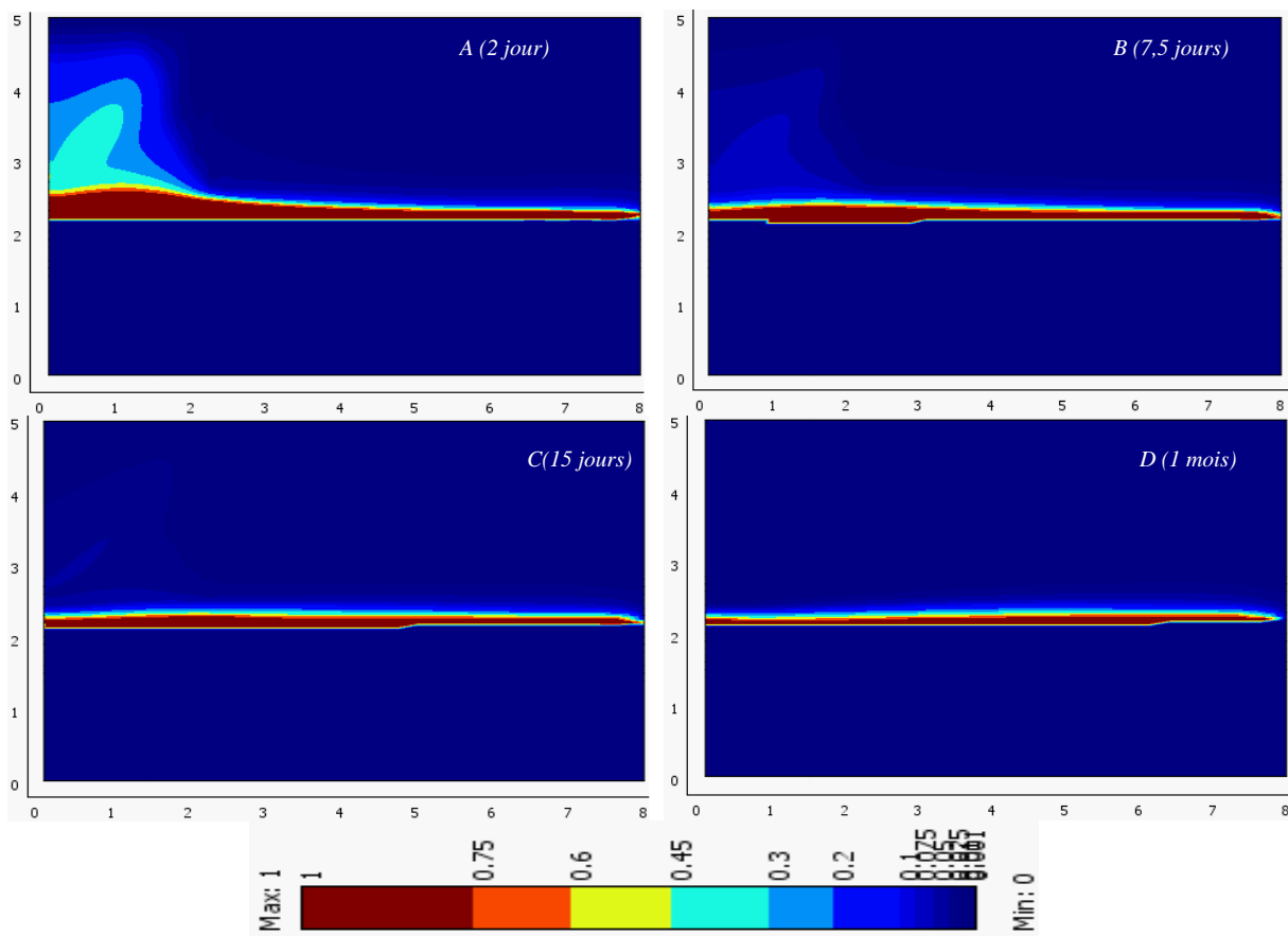
Figures V-14(A-D) : Concentration relative du polluant en phase gazeuse \left(\frac{C_{g,\beta}}{C_{g,\beta}^{sat}}\right) (étape MPE)
