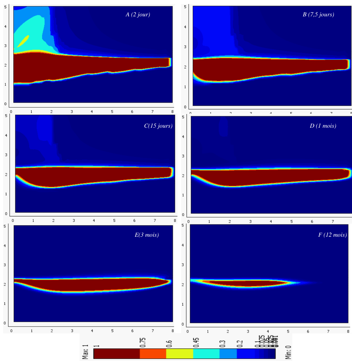
Figures V-16(A-F) : Concentration relative du polluant en phase aqueuse \left(\frac{C_{w,\beta}}{S_{w,\beta}^{eff}}\right) (étape MPE)
