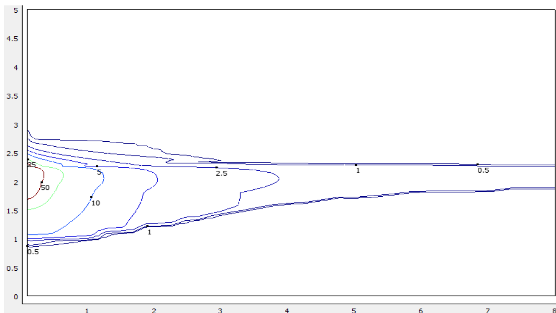
FigureV-18: Coefficient de transfert PLNA/phase aqueuse \lambda_{o-w,\beta} en [h^{-1}] à 1 journée (étape MPE)
