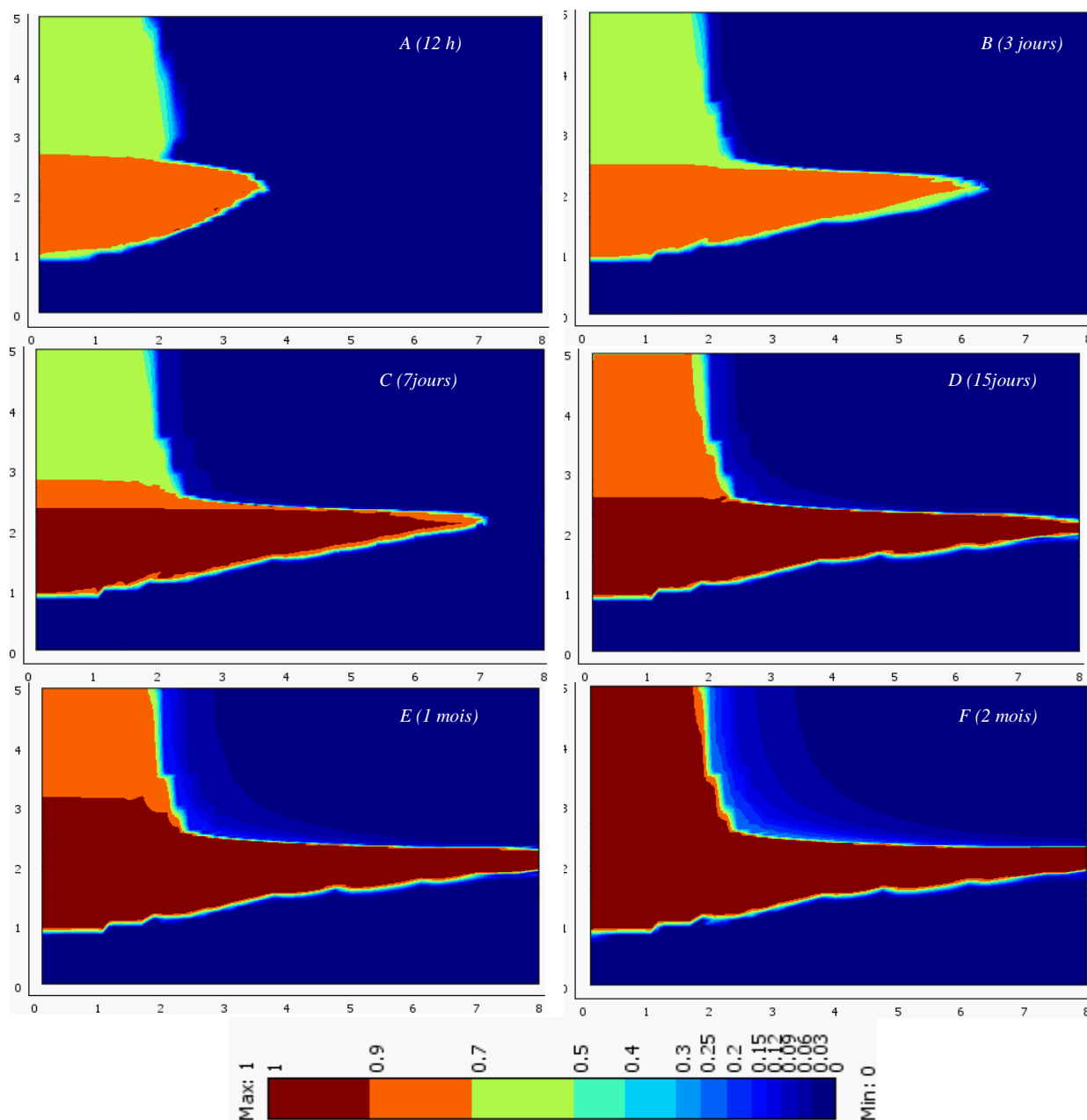
Figures V-6 (A-F) : Concentration relative du polluant en phase aqueuse \left(\frac{C_{w,\beta}}{S_{w,\beta}^{eff}}\right) (étape de propagation)
