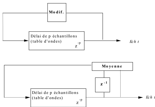
Figure 3 : l'algorithme Karplus-Strong
