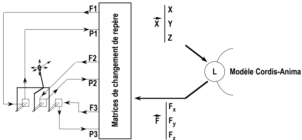
Figure 8 : communication TGR / simulation dans le cas d'une simulation 3D. La matrice de changement de repère permet de transformer les coordonnées des trois touches dues au système d'adaptation morphologique en projection suivant les 3 axes de l'espace réel.
