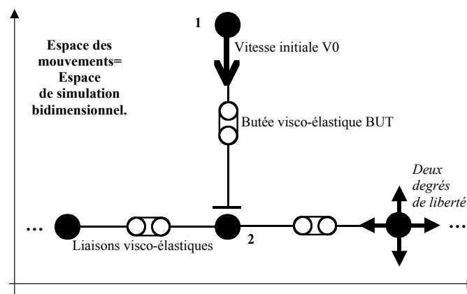
Figure 5 : modèle bidimensionnel pour une percussive élémentaire.
