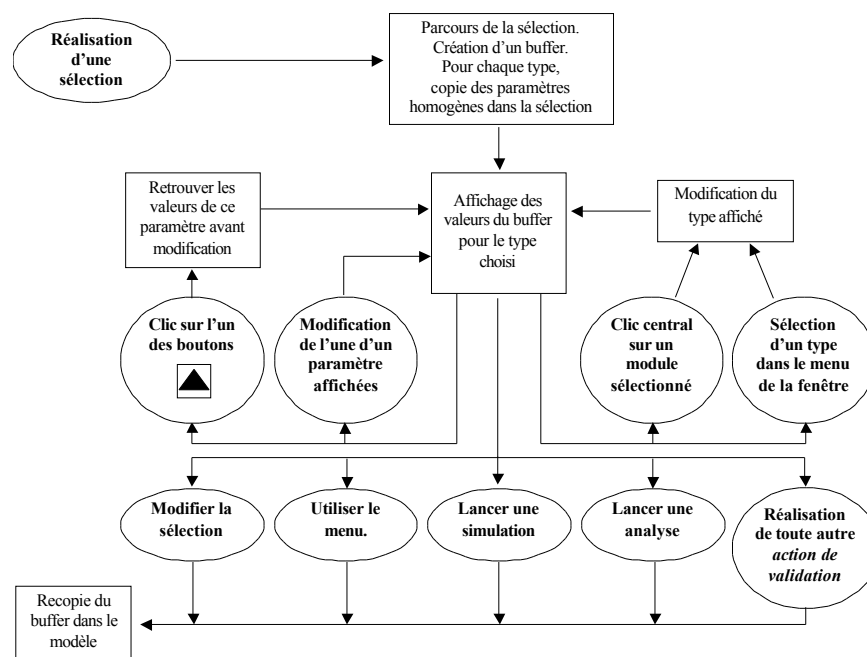
Figure 32 : flux d'interface avec la fenêtre des paramètres de GENESIS 1.3. Action de validation et validation implicite.
