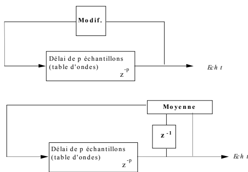
Figure 3 : l'algorithme Karplus-Strong
