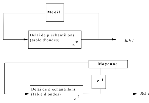
Figure 3 : l'algorithme Karplus-Strong
