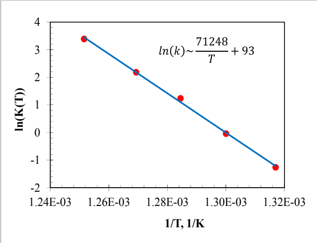
Fig. 3.1-6. Dependence of \ln(K(T)) versus 1/T .
