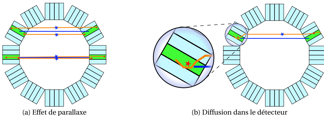
FIGURE 1.12 – En (a) la longueur des cristaux entraîne des effets de parallaxe lorsque l'on s'éloigne du centre du champ de vue. En (b) la diffusion des photons \gamma dans le détecteur peut entraîner un décalage de la LOR détectée.
