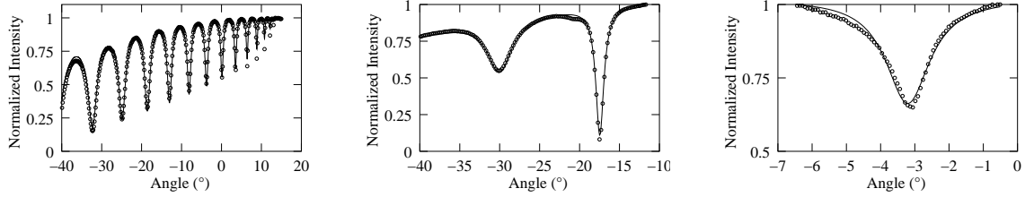
(a) Film de S1818 sur substrat de silicium (b) Film de ZnO :Al sur substrat de verre (c) Film d'ITO sur substrat de verre
