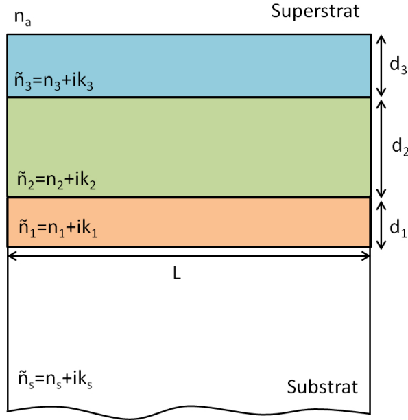
FIGURE 2.2 – Schéma de principe d'un guide d'onde à trois couches à effet EO (Pockels) en configuration de l'effet EO transversal.
