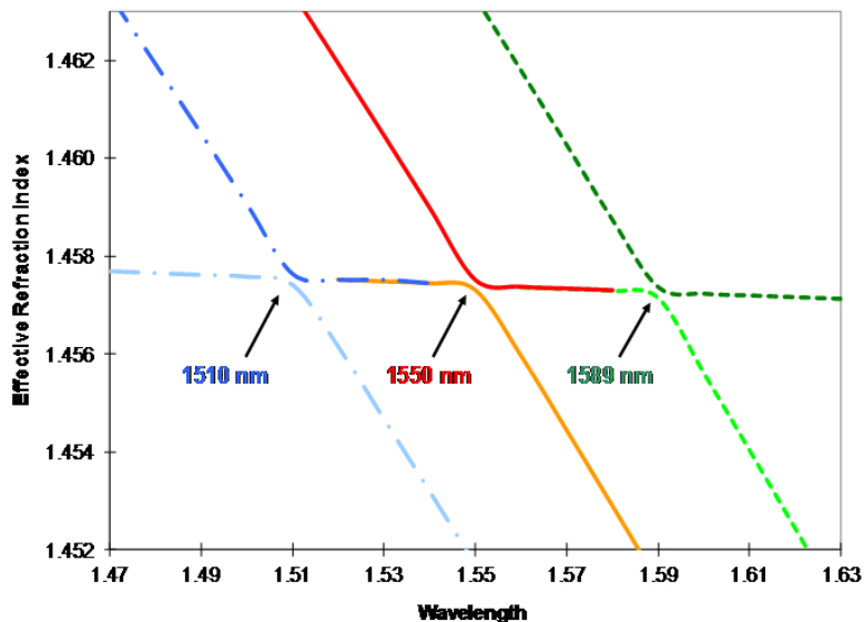
FIGURE 2.14 – Dispersion des modes du coupleur dans la plage spectrale du couplage.
