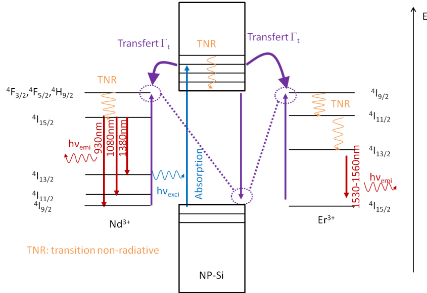
FIGURE 2.23 – Schéma de bande illustrant le couplage d'une Np-Si vers les ions Nd^{3+} et Er^{3+} .
