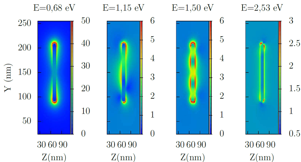
FIGURE 3.8 – Carte 2D du rapport \frac{E}{E_0} d’un nanofil d’or de rapport d’aspect R = 12 obtenue par ADE-FDTD.
