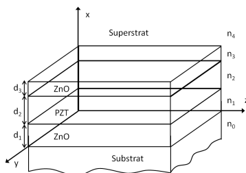
FIGURE 2.9 – Schéma d'un guide d'onde plan tricouches.
