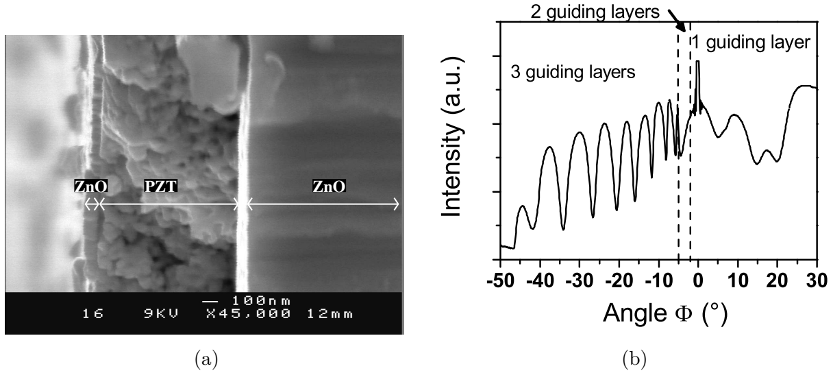
FIGURE 2.11 – (a) Image MEB d’un guide d’onde planaire à trois couches (b) Spectre M-lignes obtenu avec l’échantillon observé en MEB (figure 2.11a) mesuré à 29 mm du centre du substrat en mode TE [21]
