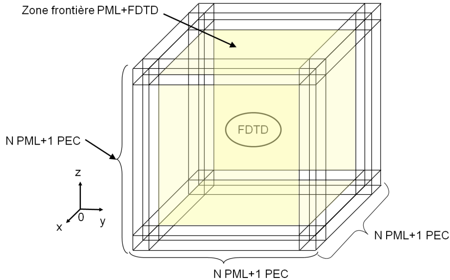
FIGURE 3.3 – Schéma en trois dimensions de la zone de calcul, qui comprend la zone FDTD entourée de N cellules de PML elle-même entourée d’une couche d’un conducteur électrique parfait [PEC : perfect electric conductor ( E=0 et H=0 )].
