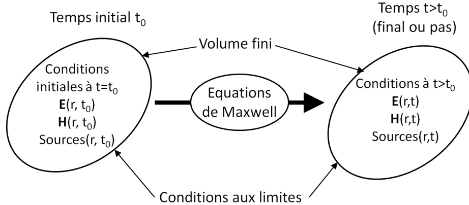
FIGURE 3.1 – Schéma de principe illustrant l'évolution dans le temps du champ électromagnétique régié par les équations de Maxwell à l'intérieur d'un domaine de l'espace délimité par les conditions aux limites et présentant des sources électromagnétiques.
