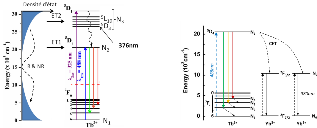
FIGURE 3.15 – Schéma de principe de l’excitation de l’ion Tb^{3+} dans les matrices de SiN_x [147] (à gauche) Description schématique des niveaux d’énergie mis en jeu dans le transfert Tb^{3+} : Yb^{3+} [148] (à droite)
