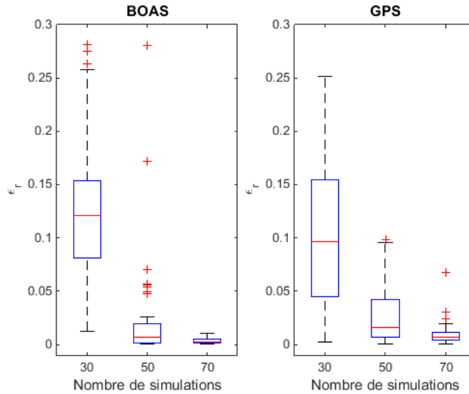
FIGURE 5.14 : Comparaison des performances des méthodes BOAS et GPS vis-à-vis de \epsilon_r avec 50 plan LHS initiaux différents pour la fonction d'Ishigami.
