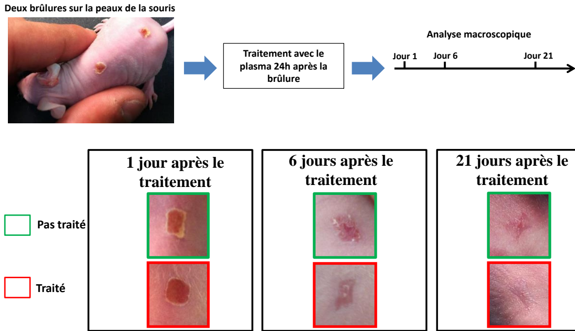
Figure 5.2. Amélioration de la procédure de cicatrisation d'une plaie causée sur la peau d'une souris, après le traitement avec des ondes d'ionisation générées en He-O 2 (99%-1%). Les images incluses dans le cadre rouge correspondent à la plaie traitée avec le plasma tandis que celles incluses dans le cadre vert représentent la plaie non traitée. Conditions : Q=2 slm, V_c=5 kV, f=10 kHz, r_c=1\% .
