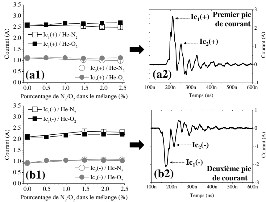
Figure 3.16. a1, b1) De valeurs I_{c1}(+)/I_{c2}(+) et I_{c1}(-)/I_{c2}(-) correspondant au premier et au deuxième pic de courant total (a2 et b2 respectivement) en fonction de mélanges He-N 2 et He-O 2 . Conditions de manip: V_p=7.3 kV, f=10 kHz, r_c=2\% , Q_{totale}=2 slm). Les points expérimentaux correspondent en deux séries de manips.
