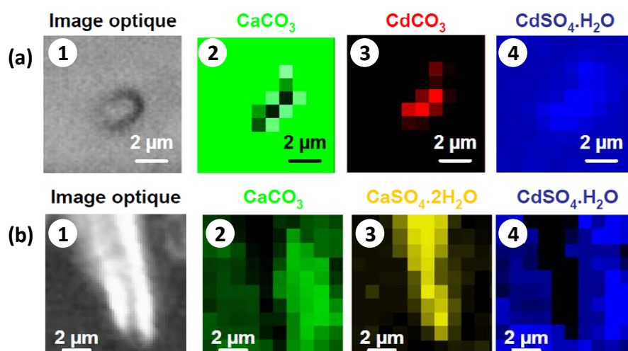
Figure 6 : (a) Images optiques (1) et Raman (2 à 4) de microcristaux de \text{CdSO}_4,8/3\text{H}_2\text{O} déposés à la surface d'un cristal de calcite après ajout d'une goutte d'eau pré équilibrée (b) Images optiques (1) et Raman (2 à 4) de la formation des sulfates de calcium et de cadmium après complète déshydratation du système (d'après Falgayrac, 2006).
