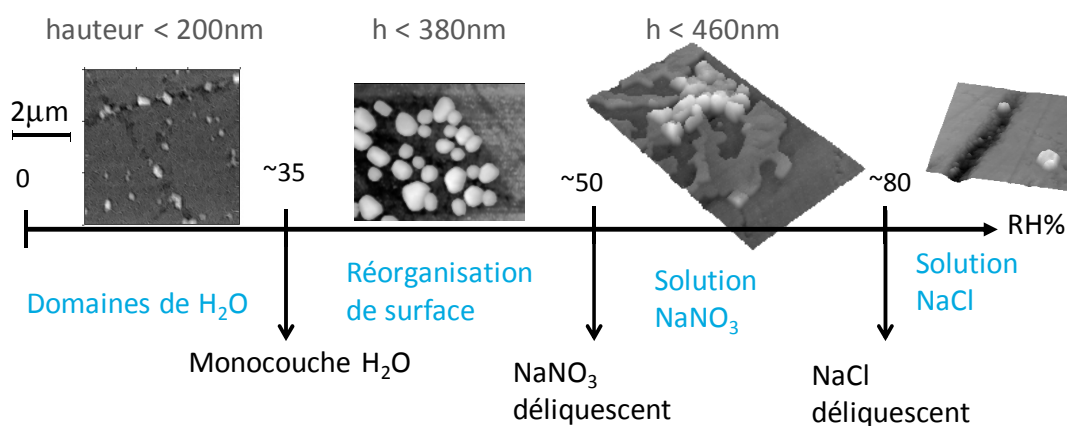
Figure 17 : Schéma représentant l'évolution de la surface de \text{NaCl}\{100\} exposée à \text{NO}_2 ( \sim 10^{15} moléc/cm 3 ) pour différentes humidités relatives. Imagerie AFM : en blanc sont représentés les îlots de \text{NaNO}_3 (avec h la hauteur des îlots), en gris la surface de \text{NaCl} .
