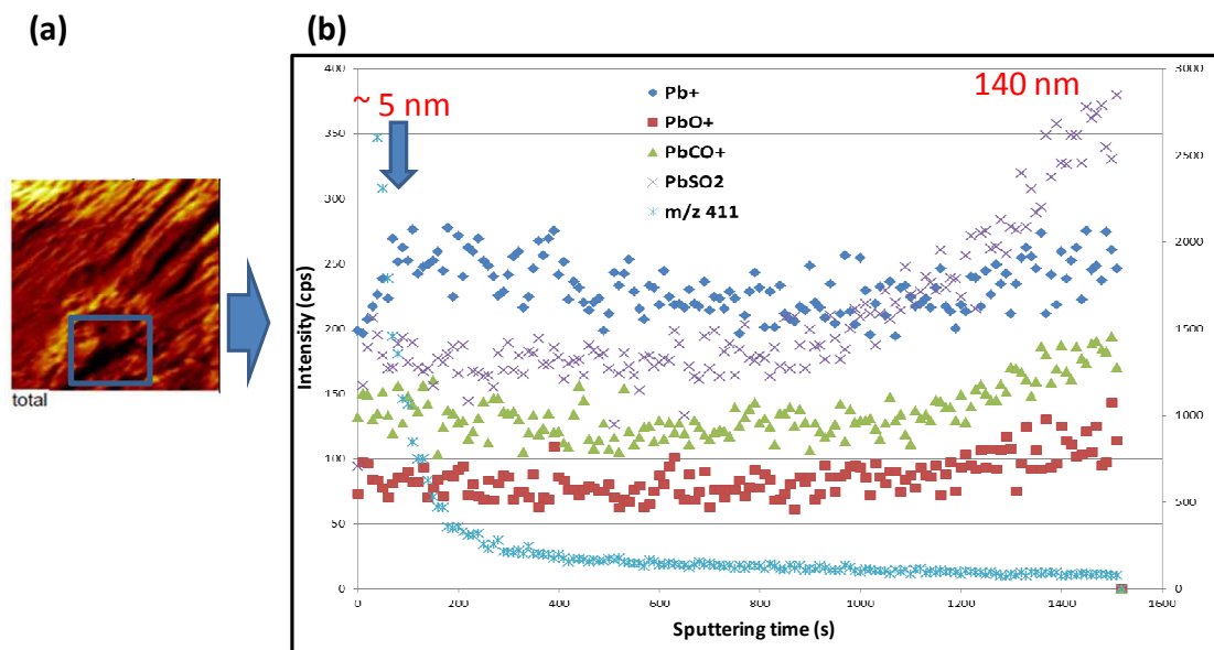
Figure 24 : Analyse en profondeur d'une zone nécrosée riche en plomb réalisée par ToF-SIMS avec une détection en mode positif (a) image ToF-SIMS (nombre de coups total) et zone abrasée (carré bleu) (b) reconstruction de l'intensité des pics de masse des fragments Pb, PbO, PbCO, PbSO 2 et m/z = 411 en fonction de la profondeur d'analyse (Schreck et al., 2012).
