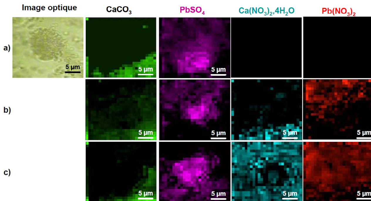
Figure 10 : Images optique et Raman de l'évolution d'un agrégat de PbSO 4 -CaCO 3 en fonction du temps d'exposition à HNO 3 (g) (2ppm, T = 20°C et HR = 40 %) ; (a) avant exposition ; (b) après 5 min d'exposition ; (c) après 35 min d'exposition.(λ = 633 nm)
