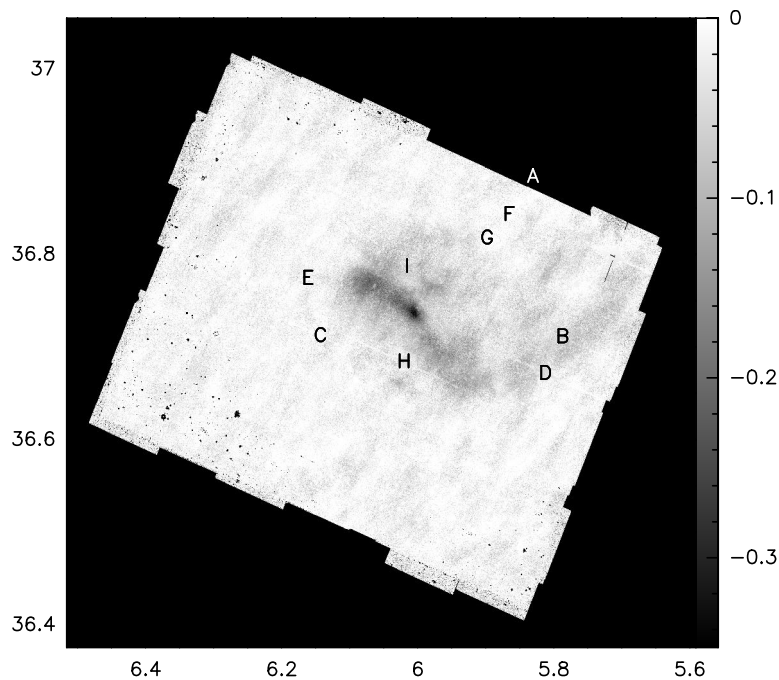
FIGURE 4.13 – Carte de l'extinction différentielle \Delta à 8\ \mu\text{m} . Les étoiles indiquées par des lettres sont celles provenant de Whittet et al. (2013) et correspondent à celles présentées Table 4.1. L'échelle est en \text{MJy sr}^{-1} .
