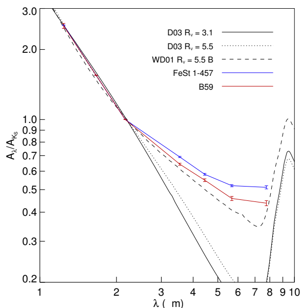
FIGURE 4.10 – Extinctions obtenues pour les nuages moléculaires denses FeSt 1–457 (en bleu) et Barnard 59 (en rouge). L'extinction des modèles de poussière de Draine (2003) et Weingartner et Draine (2001) est également représentée. On constate que le modèle WD01 5.5B est plus proche des observations et qu'aux longueurs d'onde proche-infrarouge la réponse varie peu suivant les modèles de poussière avec cette normalisation. Figure extraite de l'article d'Ascenso et al. (2013).
