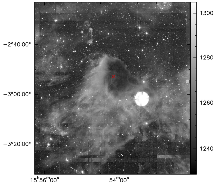
FIGURE 4.1 – L183 vu en bande R par la caméra MegaCam du Canada France Hawaiï Telescope (CFHT) . L'échelle d'intensité est en \text{Jy.sr}^{-1} . La croix rouge marque la position du cœur préstellaire.
