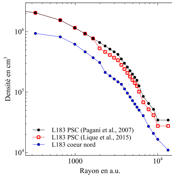
FIGURE 4.6 – Profil de densité des cœurs central (PSC) et nord (+30'', +210'' par rapport au PSC) de L183. Le profil en noir est extrait du meilleur modèle de Pagani et al. (2007). Le profil en rouge est notre interprétation de l'impact des corrections à apporter à Pagani et al. (2007) en intégrant les nouveaux coefficients de collision de \text{N}_2\text{H}^+ calculés par Lique et al. (2015). Le profil en bleu est une estimation de la densité dans le cœur nord en calquant l'apparence du profil de densité sur celui du cœur central.
