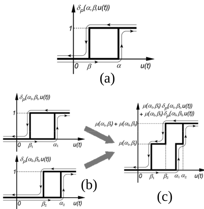
FIGURE B.1: Modélisation de l'hystérésis avec des hystérons de l'approche Preisach [144]. (a) illustration de l'hystéron, (b) deux hystérons combinés pour former la courbe d'hystérésis représentée à (c).
