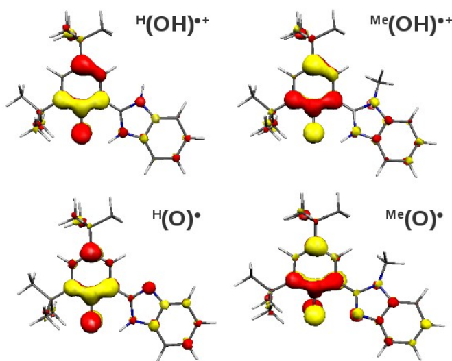
Figure 13. Structures électroniques des composés modèles du radical tyrosyle.
