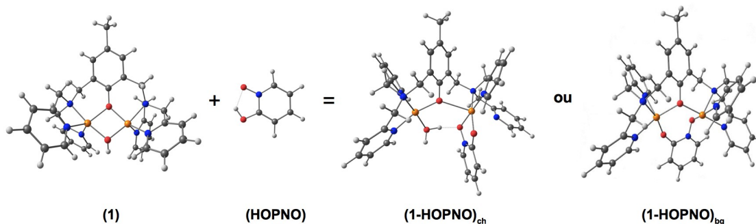
Figure 4. Illustration des modes de fixation chélatant et pontant.
