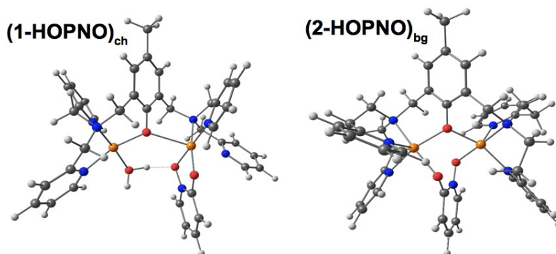
Figure 5. Modes de fixation de HOPNO au site dinucléaire à cuivre.
