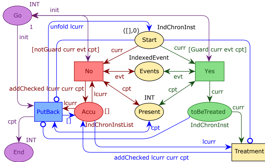
FIGURE 4.18 – Le réseau séparateur de jetons
