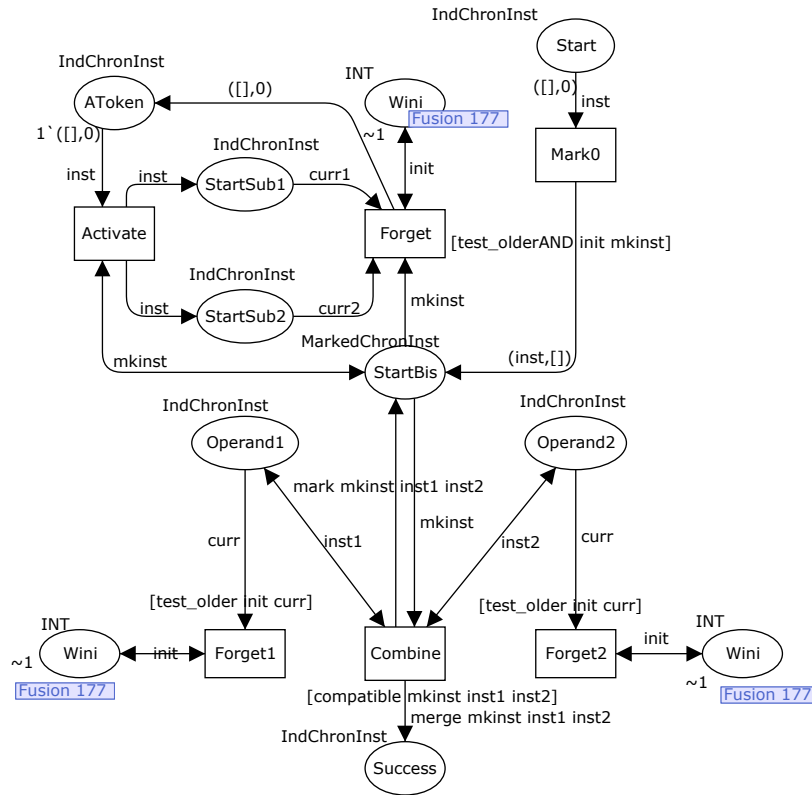
FIGURE 4.5 – Opérateur AND
