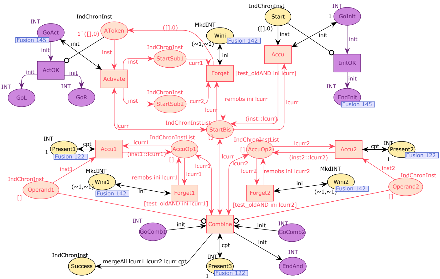
FIGURE 4.16 – Opérateur AND
