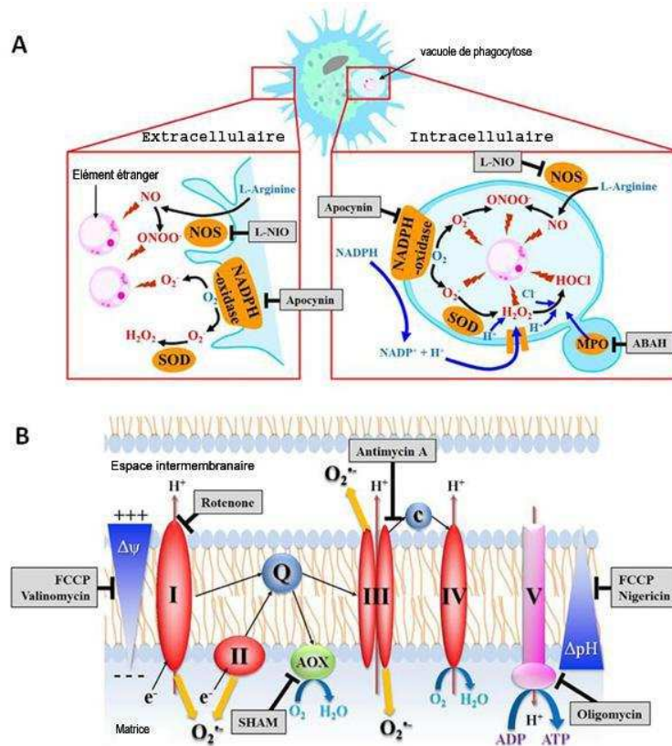
Figure 10. Espèces réactives de l'oxygène et de l'azote produites chez les hémocytes de bivalves. A. Production des ROS/RNS à la membrane plasmique (droite) et à l'intérieur du phagosome (gauche). B. Chaîne respiratoire mitochondriale hypothétique. Les inhibiteurs des molécules cibles sont indiqués en gris. SOD : superoxyde dismutase, NOS : oxyde nitrique synthase, MPO : myéloperoxydase. D'après Donaghy et al., 2012.
