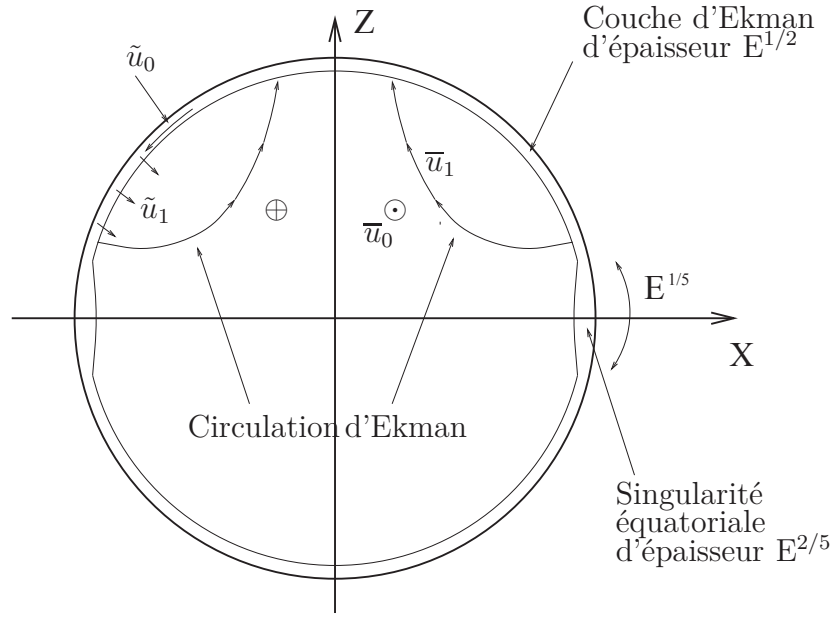
FIGURE 1.3 – Représentation schématique de l'écoulement de spin-up d'un fluide au sein d'une sphère. \bar{u}_0 est l'écoulement géostrophique azimuthal; \tilde{u}_0 la composante méridienne de l'écoulement dans la couche d'Ekman et \tilde{u}_1 le pompage d'Ekman générant la circulation d'Ekman \bar{u}_1 (Rieutord, 2014).
