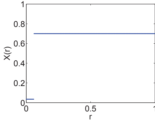
FIGURE B.1 – Profil d'abondance en hydrogène en fonction du rayon adimensionné d'un modèle ESTER dont X_0 = 0.7 , X_c = 0.05 et r_c = 6\% .
