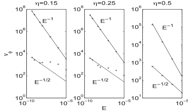
FIGURE 3.9 – Logarithme de la valeur absolue de l’amplitude de la vitesse azimutale numérique en fonction du logarithme du nombre d’Ekman à z = 0.5 . À gauche : \eta = 0.15 , au milieu : \eta = 0.25 , à droite : \eta = 0.5 . Dans le cylindre tangent, les points de mesures sont respectivement s = 0.1, 0.2, 0.25 , la vitesse azimutale suit une loi d’échelle en E^{-1/2} . Elle est proportionnelle à E^{-1} dans l’enveloppe (point de mesure s = 0.65 ). La vitesse azimutale est principalement négative pour les “petits” cœurs (e.g. \eta = 0.15 ou \eta = 0.25 ) et positive quand le cœur est plus gros (e.g. \eta = 0.5 ).
