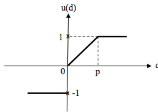
Figure 29. Fonction d'utilité
