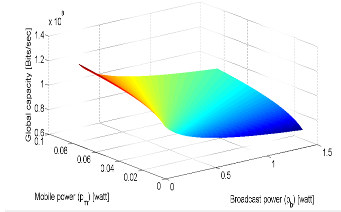
FIGURE 9 – Capacité globale (bits/sec) en fonction de p_b et p_m , mode 8K du DVB, bande recouverte = 7.61 MHz, d=100\text{m} .
